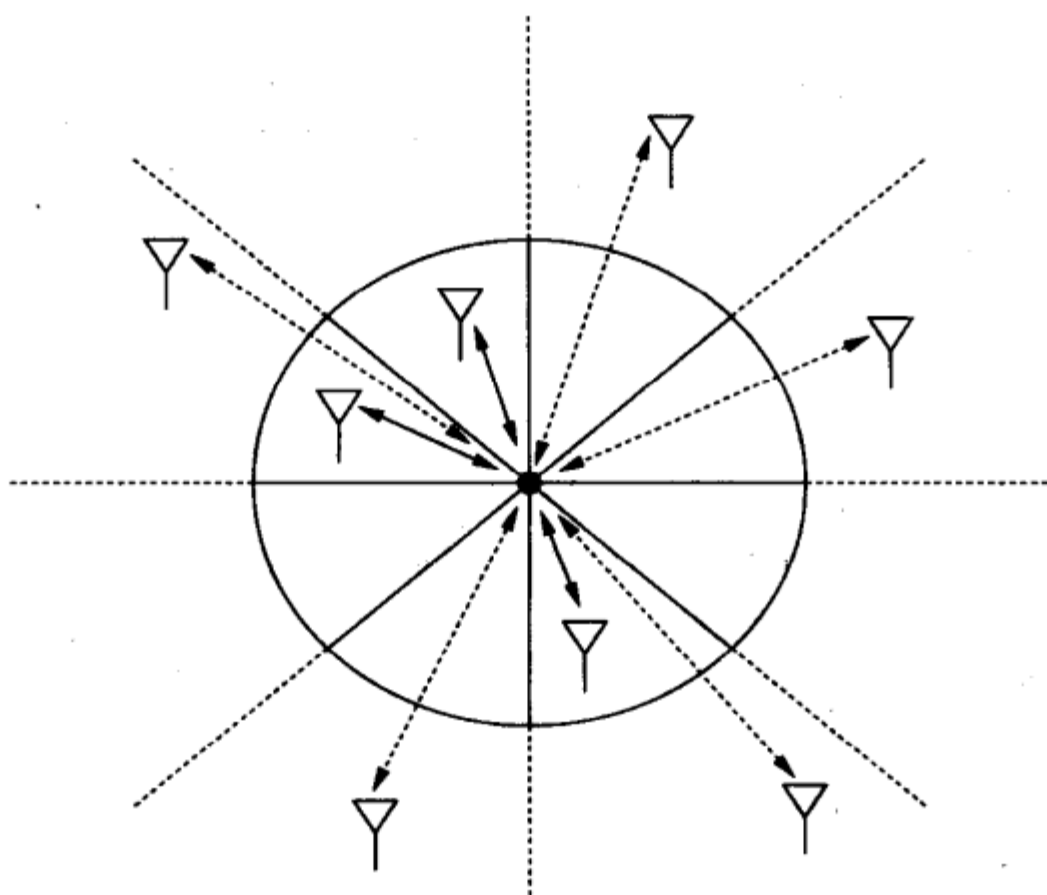
图15-8 N=8 时圆形小区的扇区化
