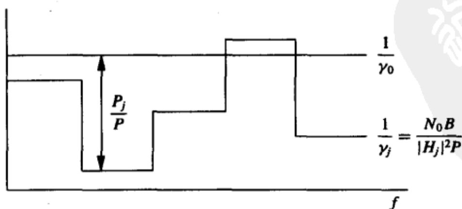
图4-11 分块频率选择信道的注水法功控
