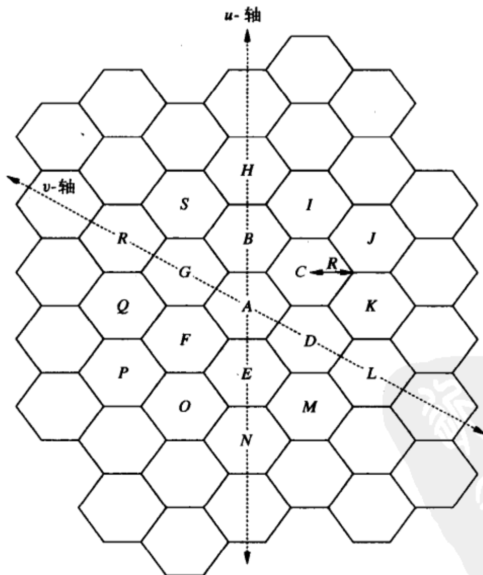
图15-4 正六边形小区复用距离坐标图
