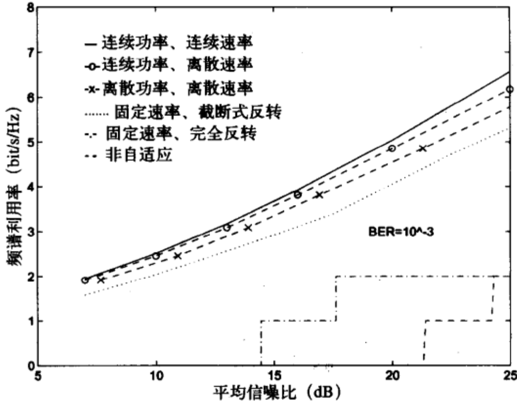
图9-7 对数正态阴影下的频谱利用率 ( \sigma_{\nu_{dB}} = 8\text{dB} )
