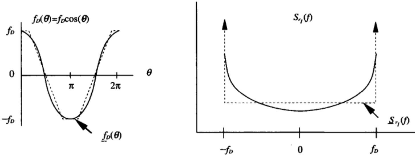
图3-7 余弦函数及功率谱密度的折线近似
