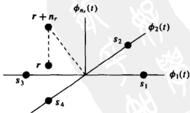
图5-5 接收信号投影为接收向量 r
