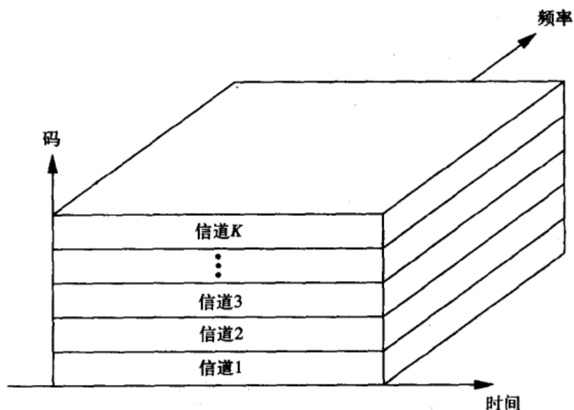
图14-4 码分多址
