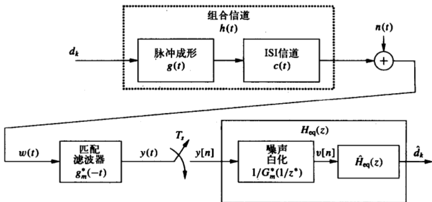
图11-4 带有噪声白化滤波的MMSE均衡
