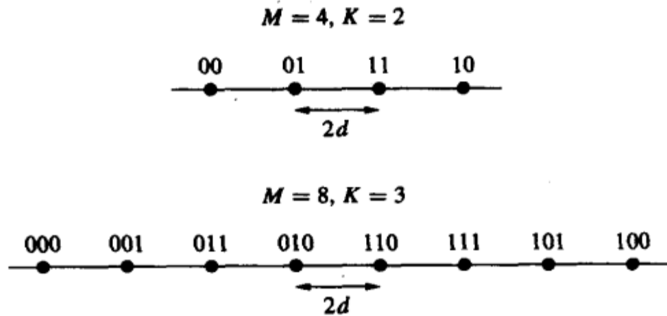
图5-12 MPAM星座的格雷码
