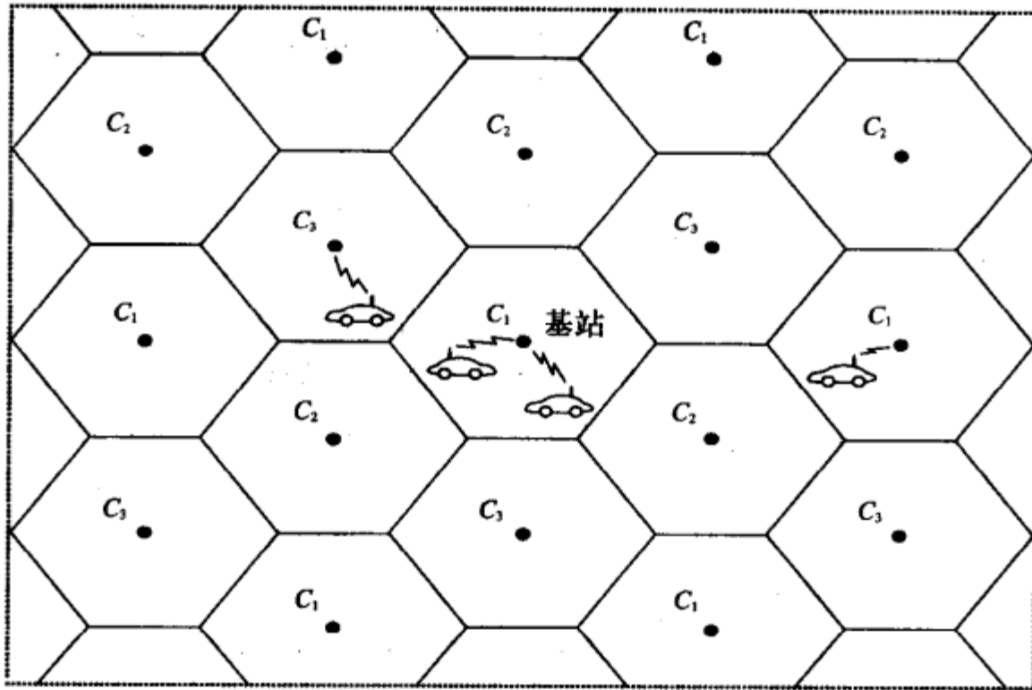
图15-1 蜂窝系统
