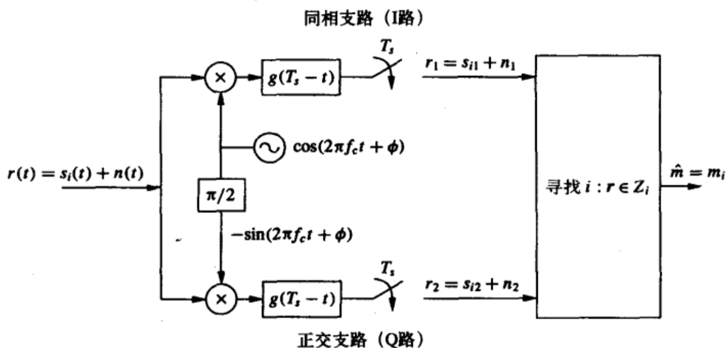
图5-11 幅度/相位解调器(相干: \phi = \phi_0 )
