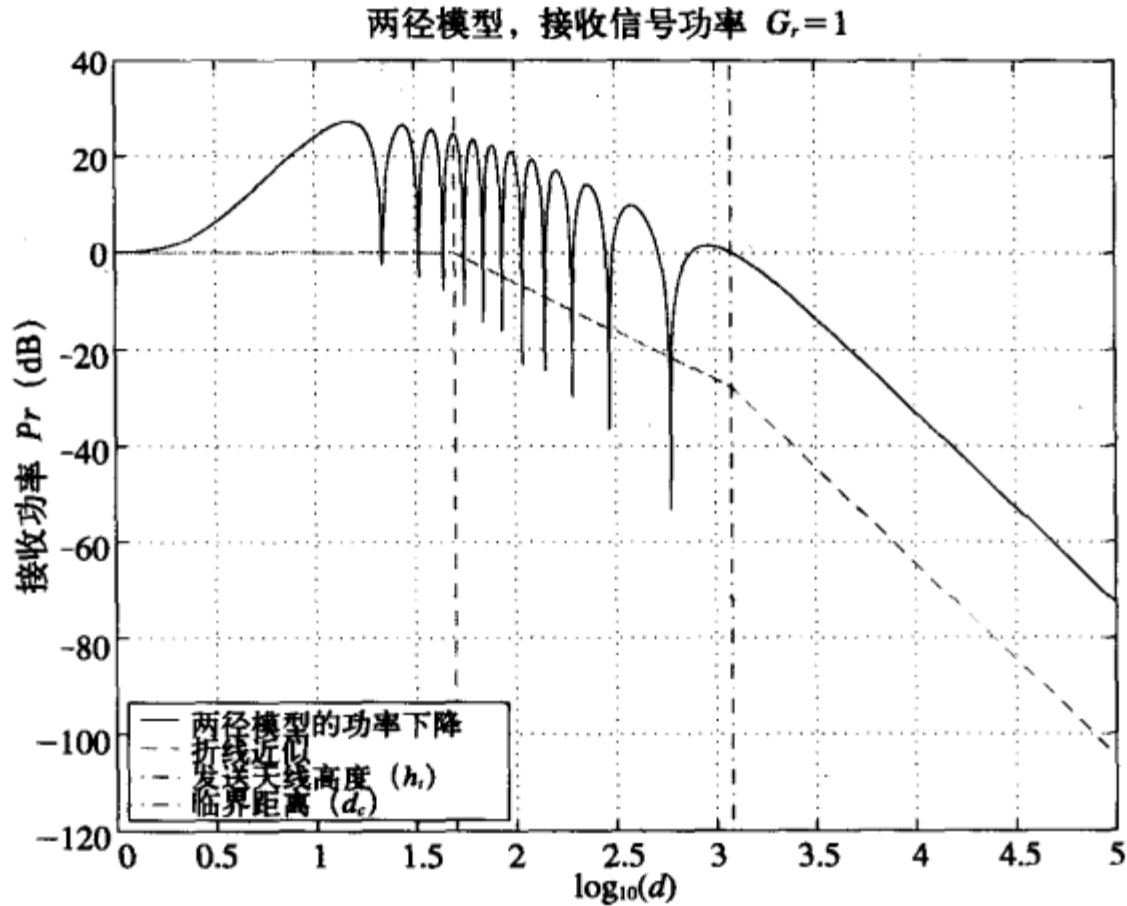
图2-5 两径模型中接收功率与距离的关系
