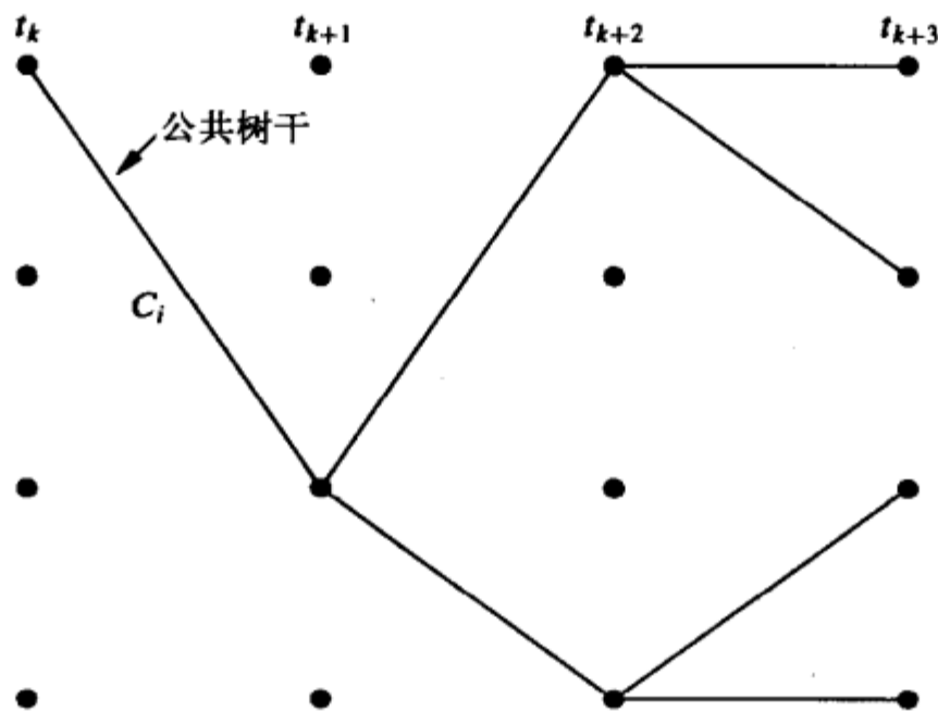
图8-9 所有幸存路径的公共树干
