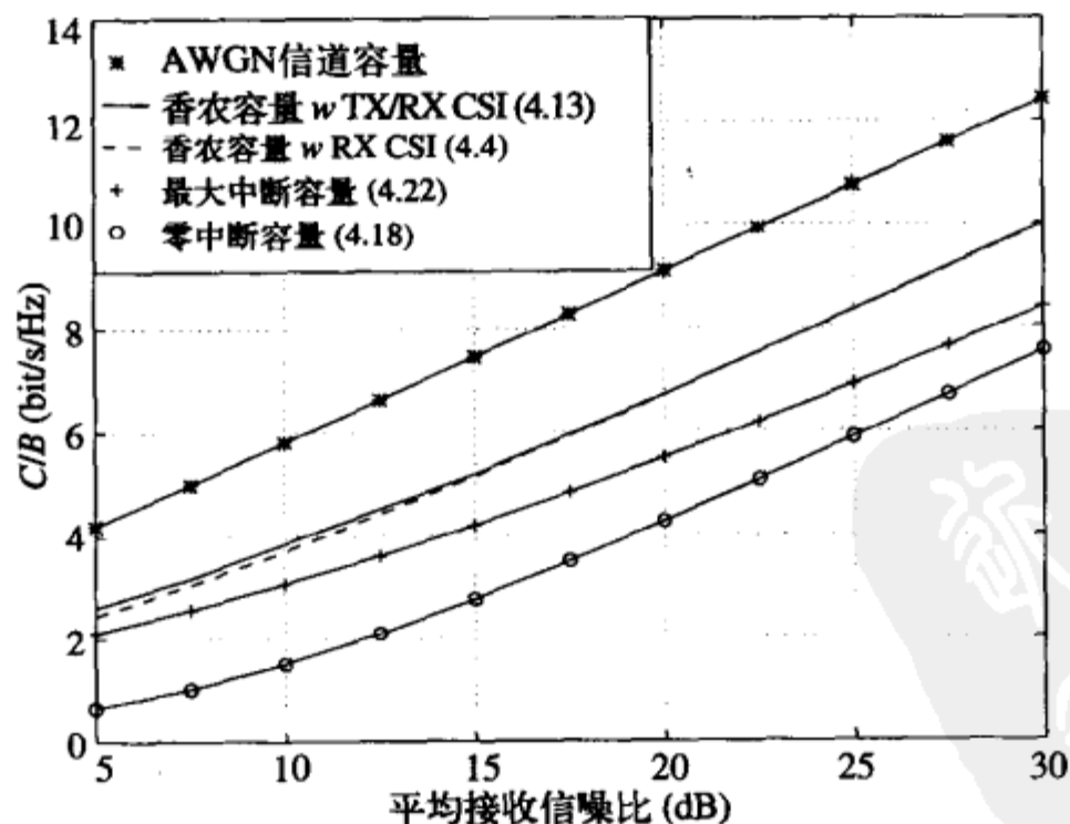
图4-6 对数正态衰落下的信道容量
