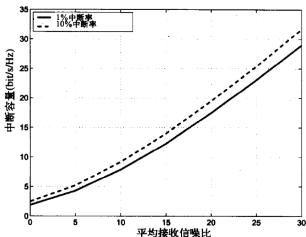
图10-5 4 \times 4 MIMO信道的中断容量
