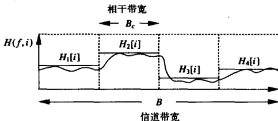
图4-12 频率选择性衰落下的信道划分
