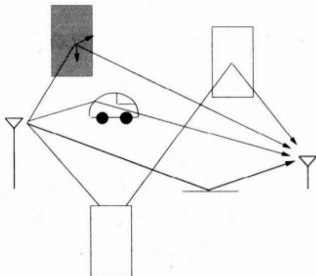
图2-3 反射、绕射与散射分量
