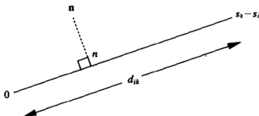
图5-9 噪声投影
