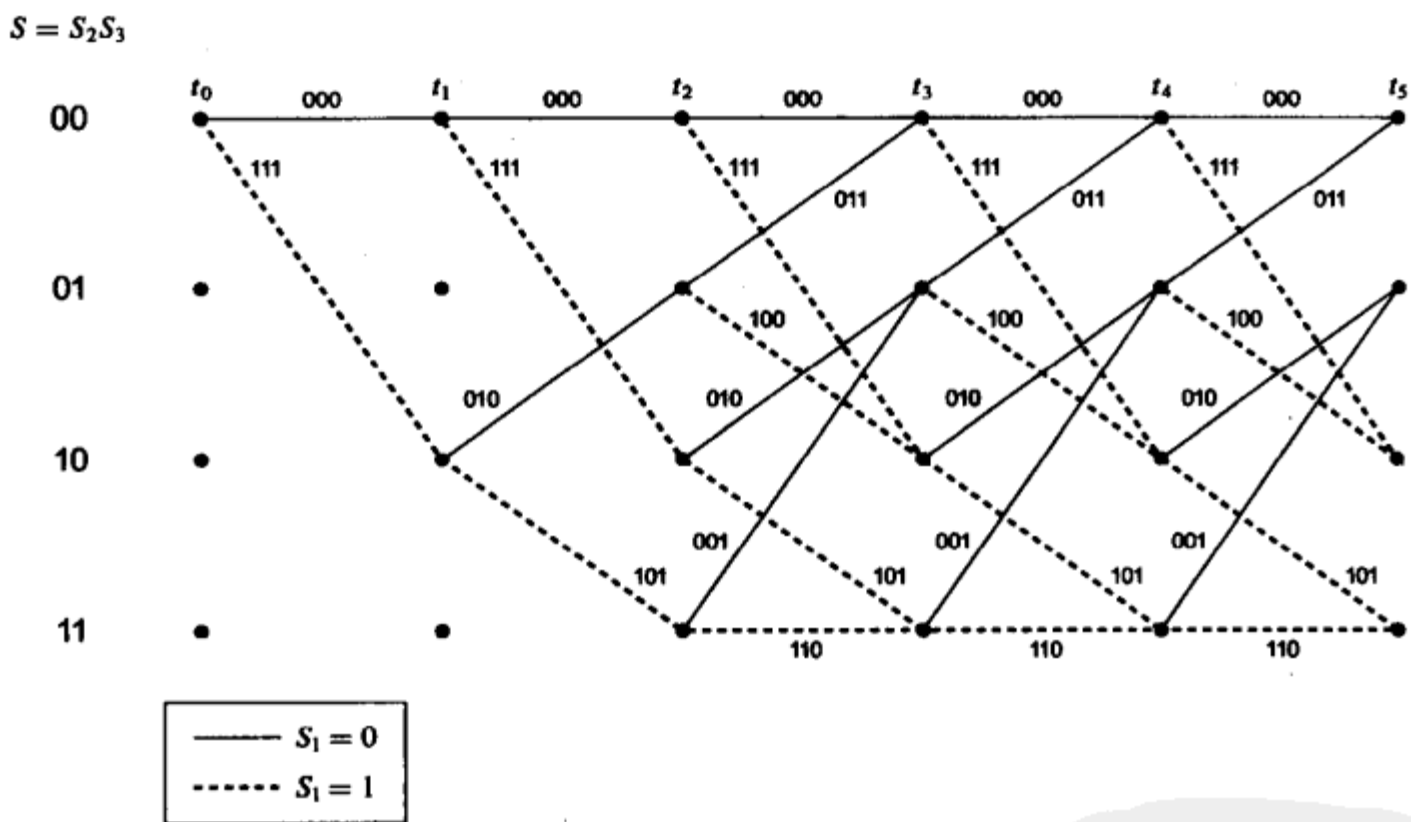
图8-7 格图
