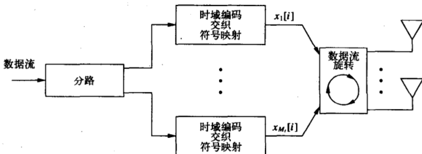
图10-12 带有数据流旋转的对角编码
