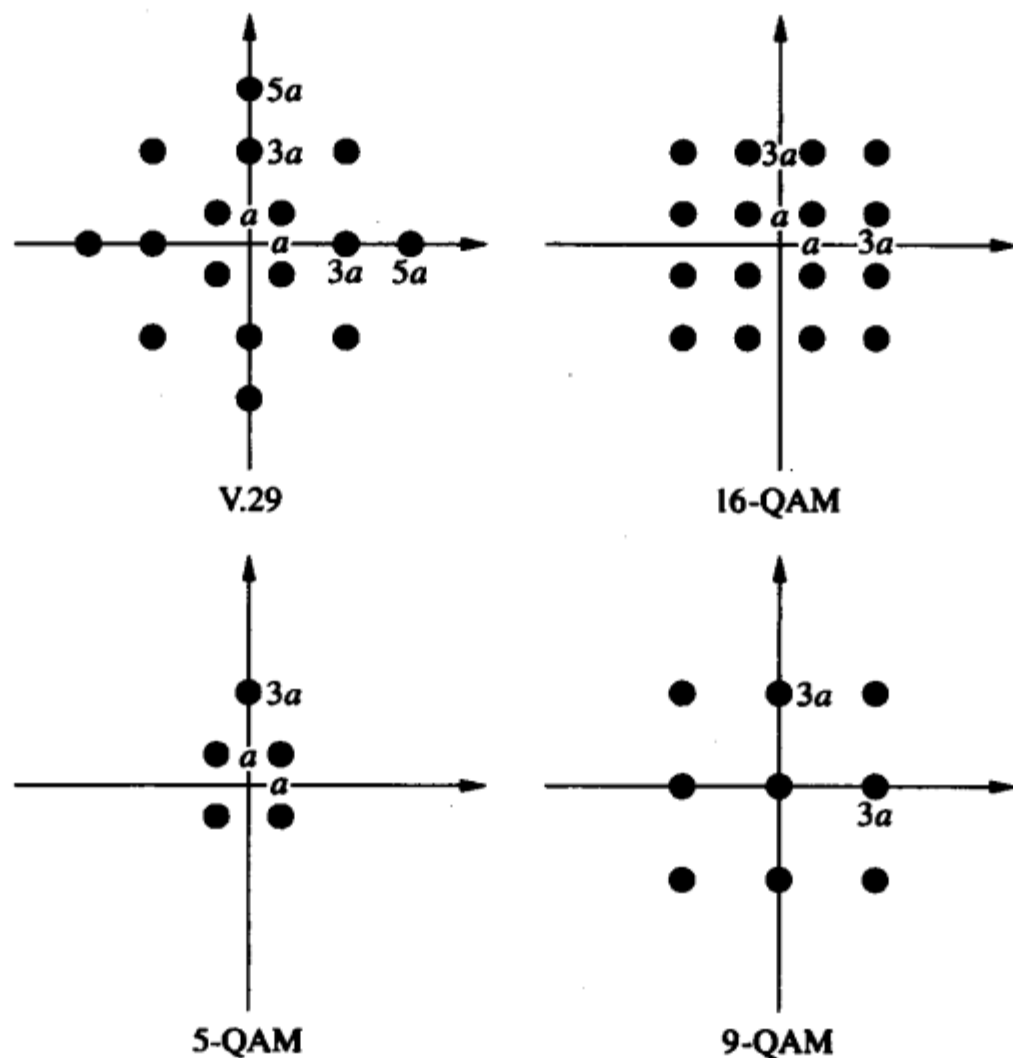
图6-7 题6.5的星座图
