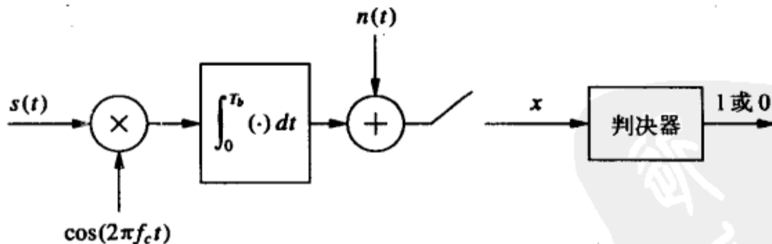
图6-6 题6.4的BPSK解调器
