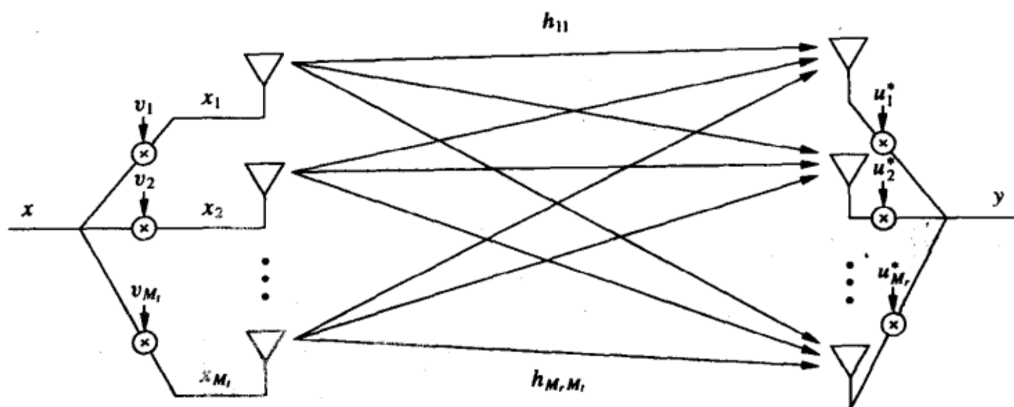
图10-7 波束成形的MIMO信道
