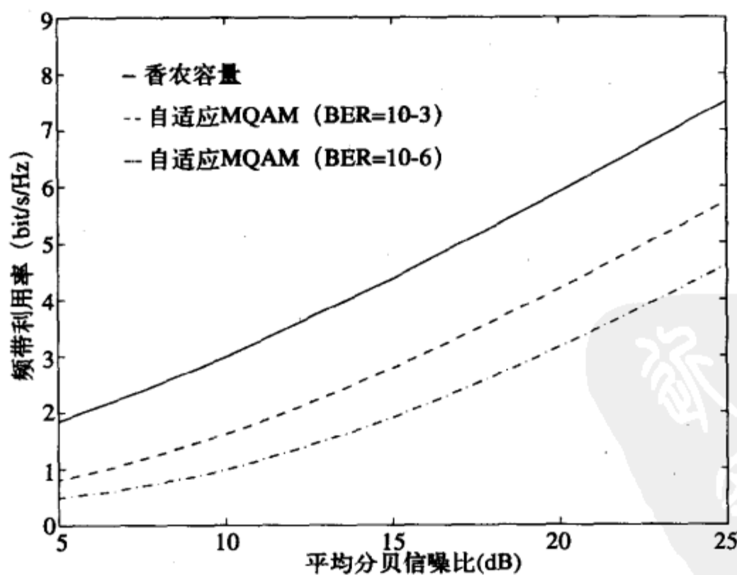
图9-3 瑞利衰落下的平均频带利用率
