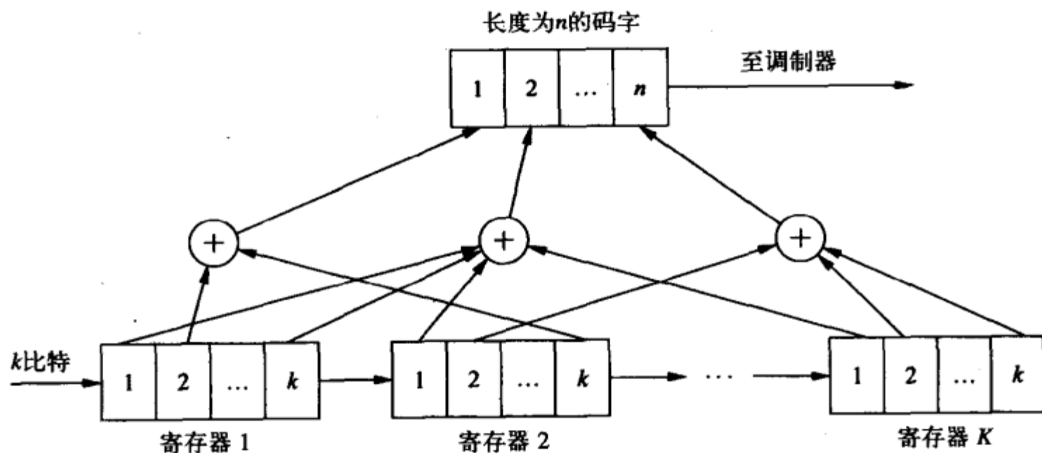
图8-5 卷积码编码器
