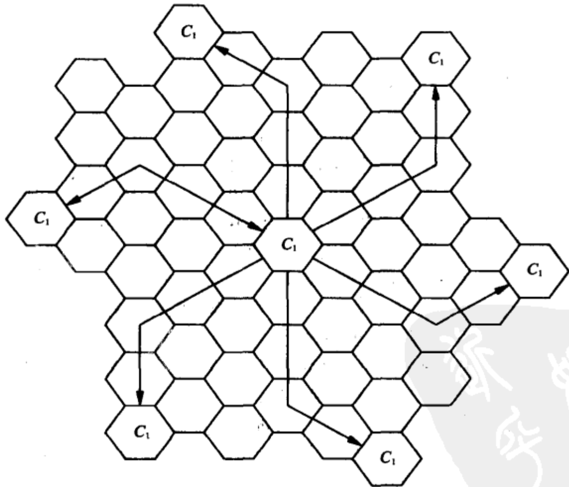
图15-6 正六边形小区的信道分配
