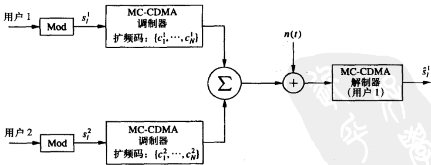
图13-18 两用户的多载波CDMA系统
