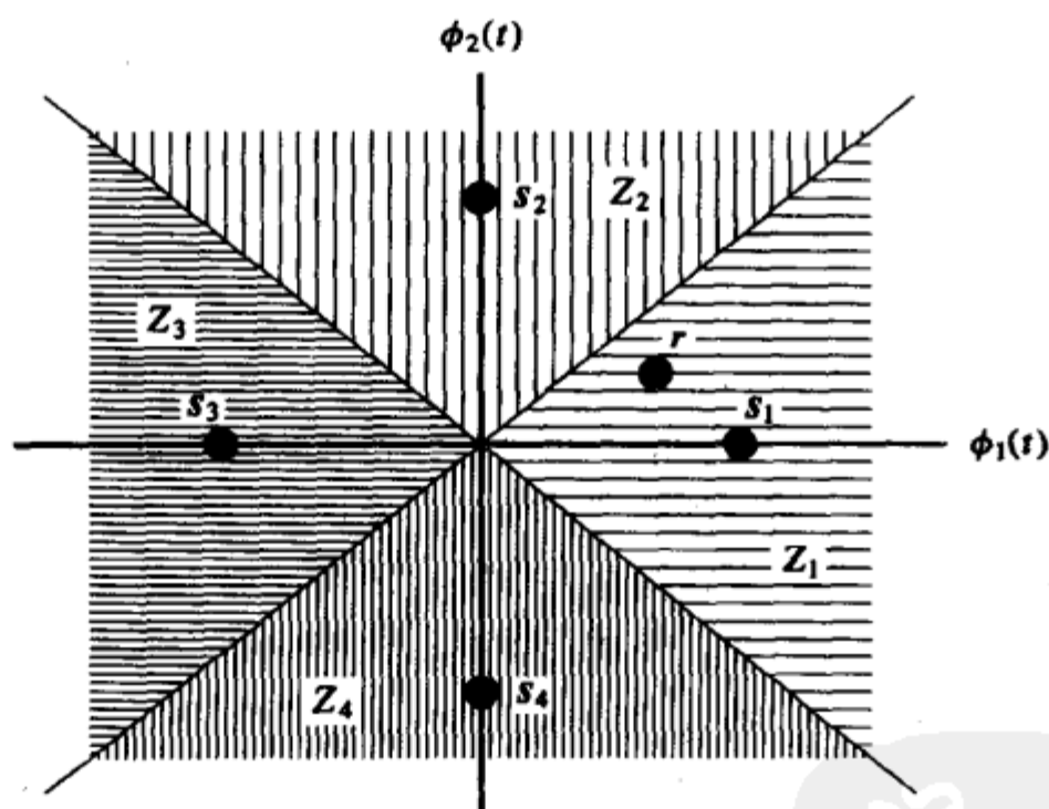
图 5-6 判决域
