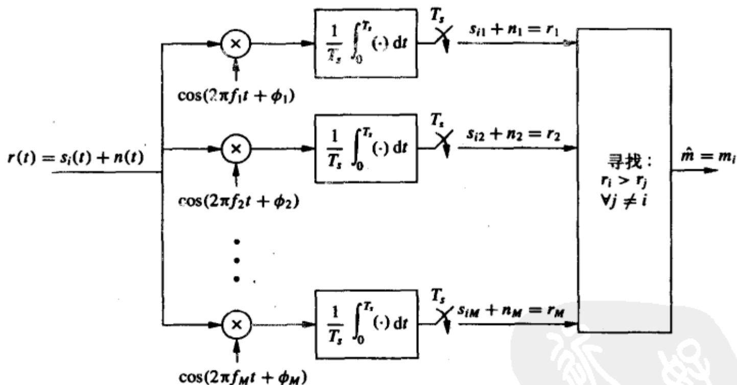
图5-23 频率解调器(相干)
