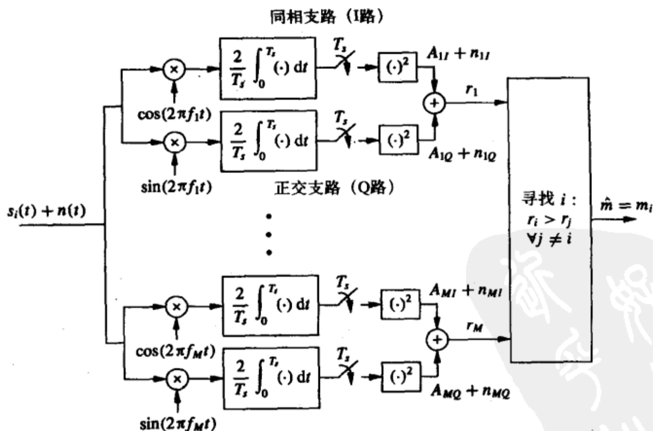
图5-25 非相干FSK解调
