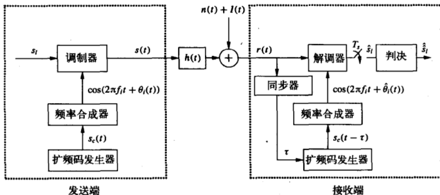
图13-11 FHSS系统模型
