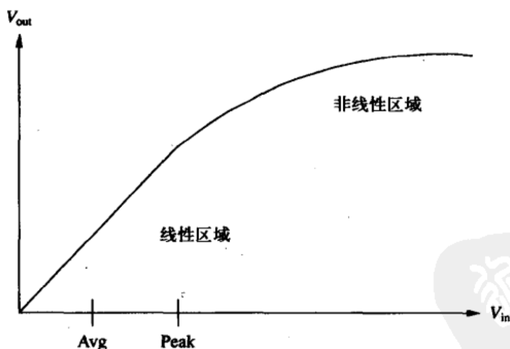
图12-11 典型功放的特性
