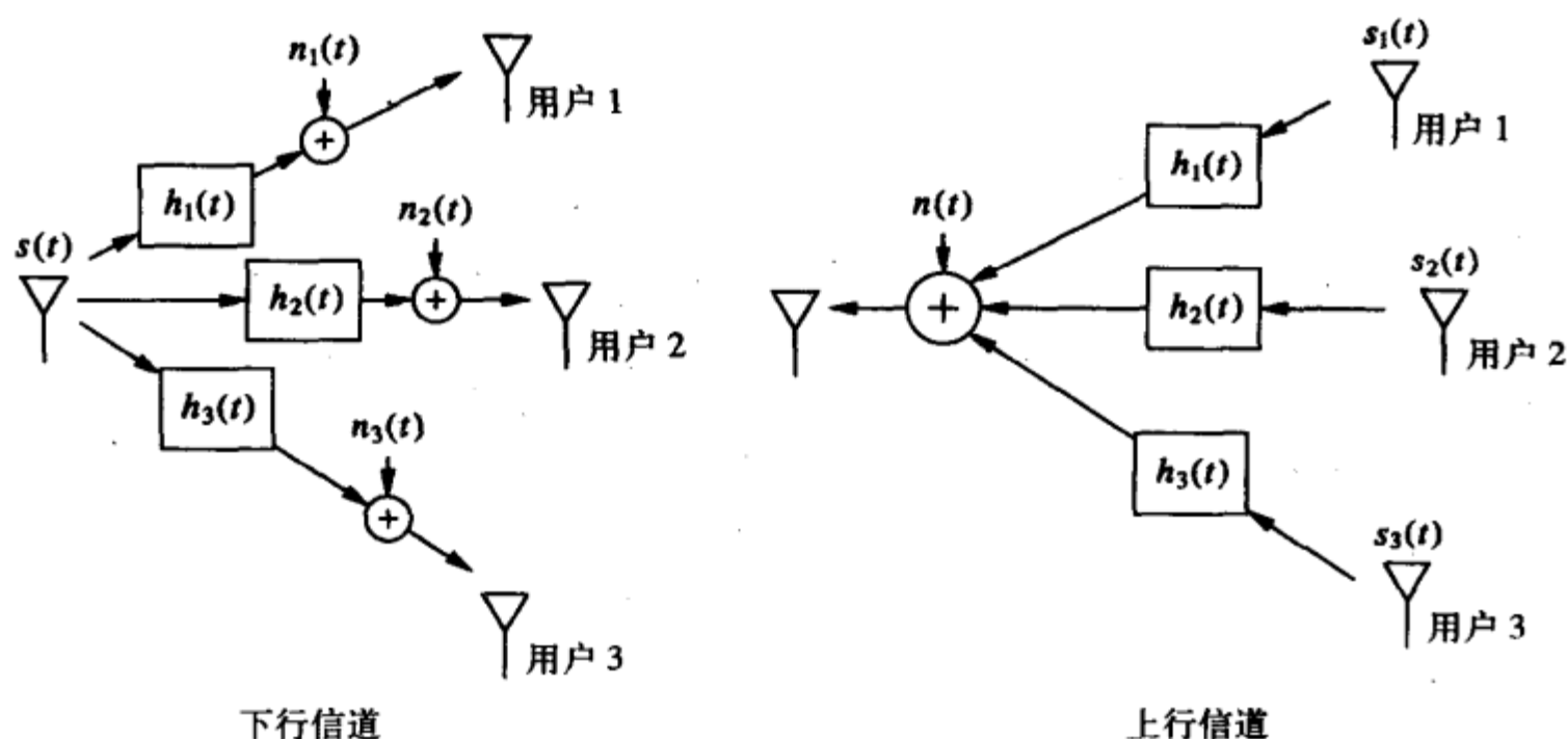
图14-1 下行信道和上行信道
