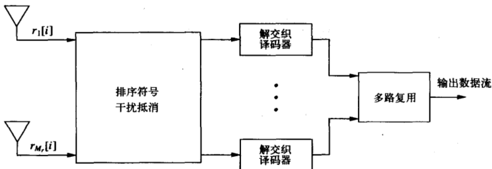
图10-11 线性复杂度的V-BLAST接收机
