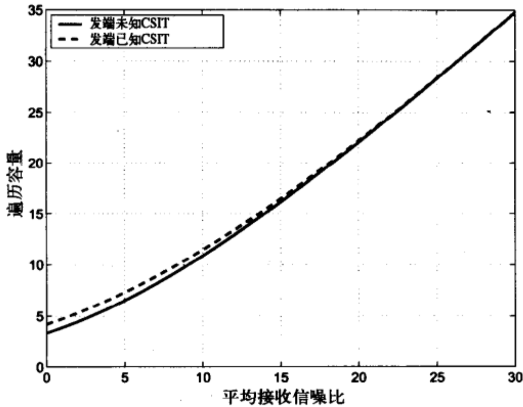
图10-4 4 \times 4 MIMO信道的遍历容量
