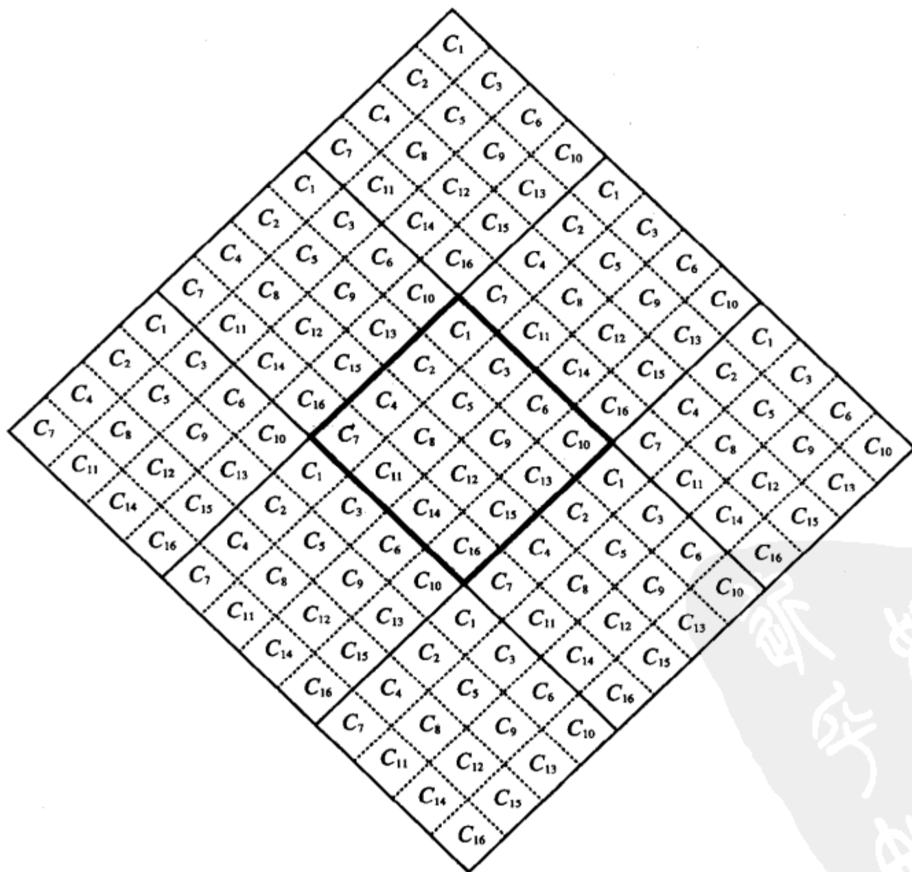
图15-5 菱形小区的小区簇
