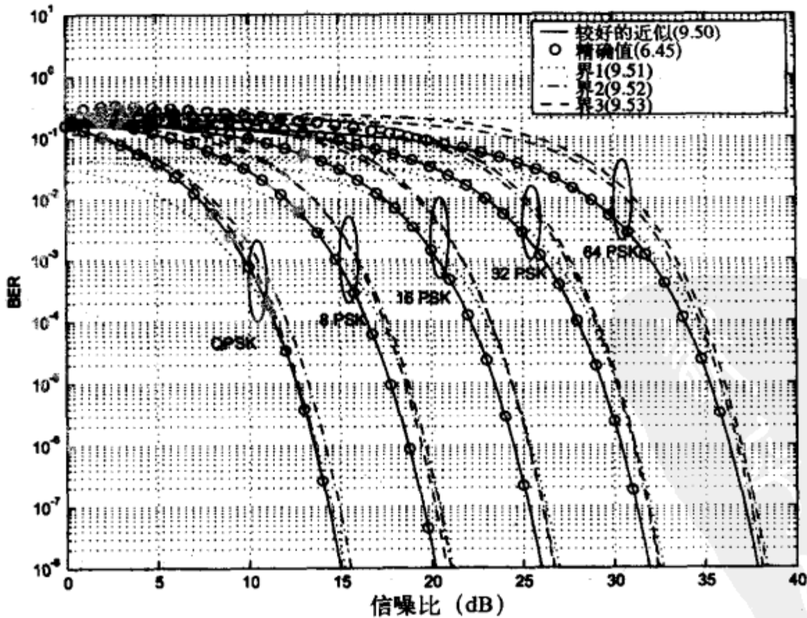
图9-14 MPSK的误比特率界
