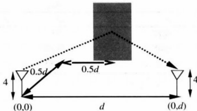
图2-11 题2.11中带散射的系统
