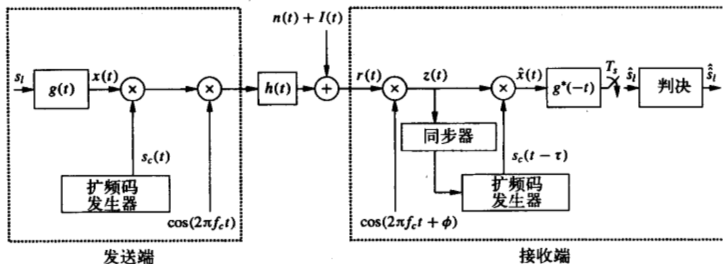
图13-5 DSSS系统模型
