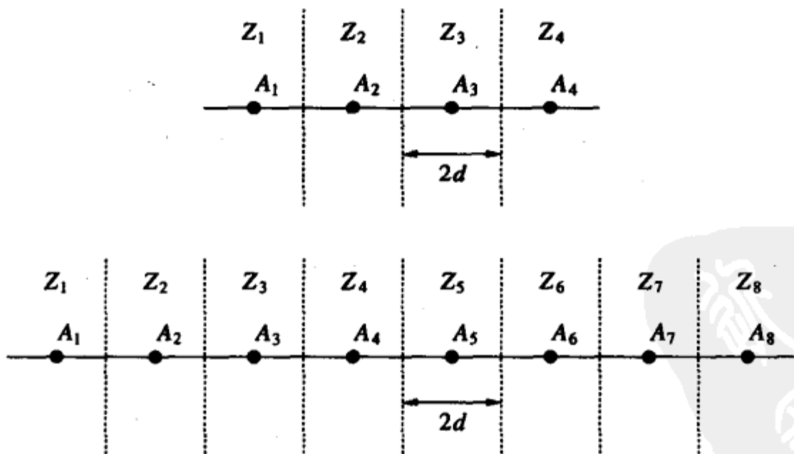
图5-13 MPAM的判决域
