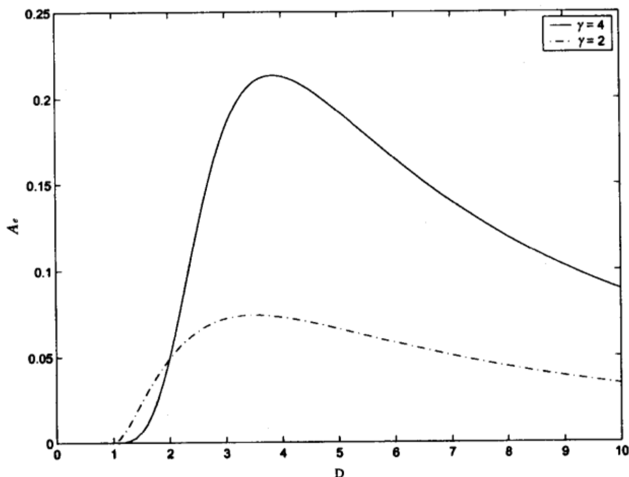
图15-10 AWGN上行链路的面积频谱效率 ( \gamma = 2 和4)
