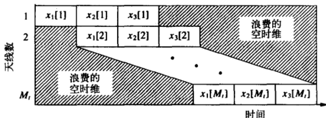
图10-13 数据流旋转
