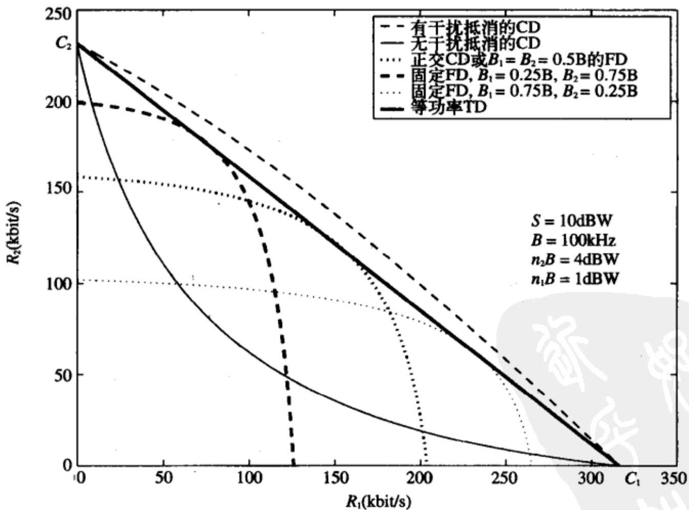
图14-10 两用户信噪比相差3dB时的容量域
