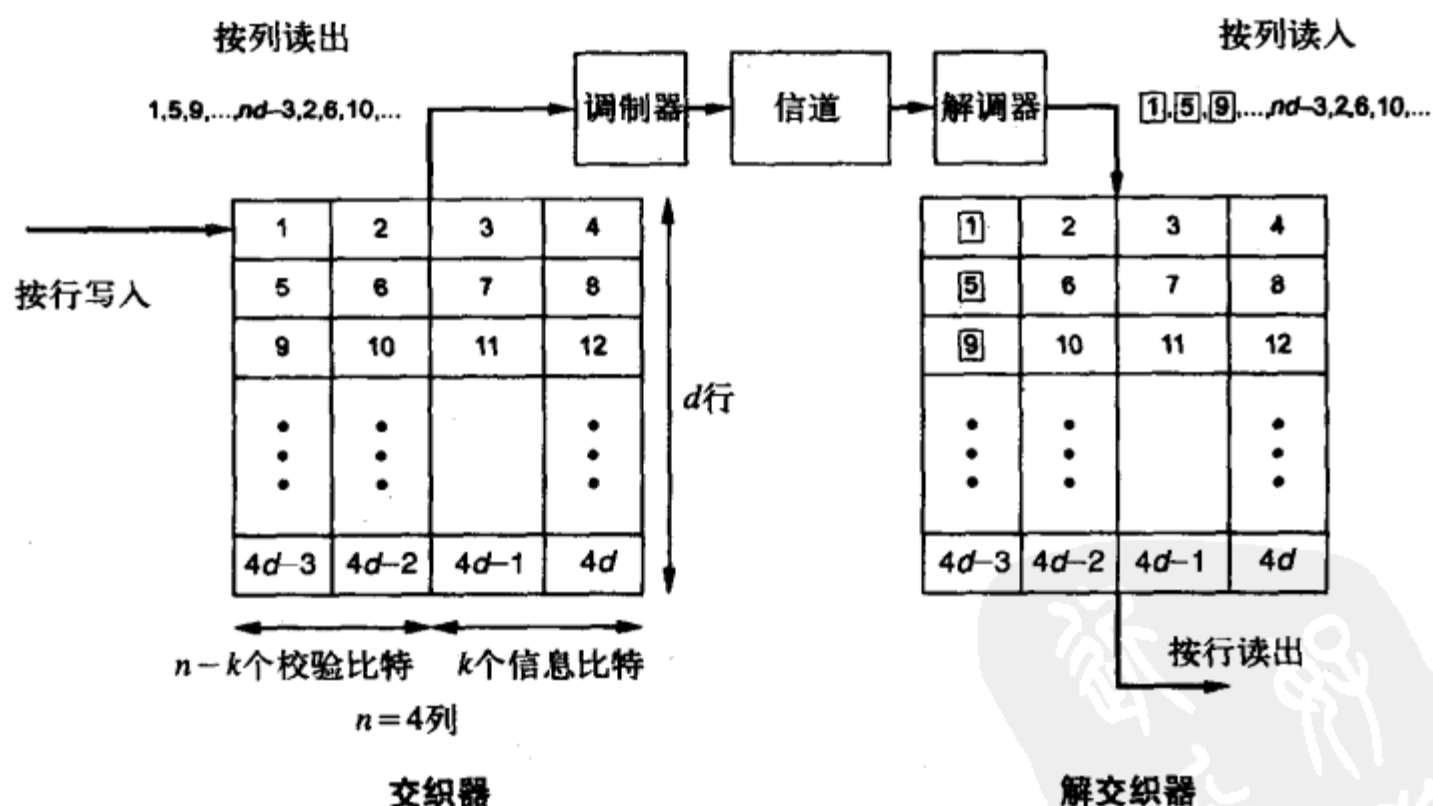
图8-19 交织/解交织
