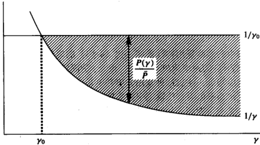
图4-5 最佳功率分配:注水法
