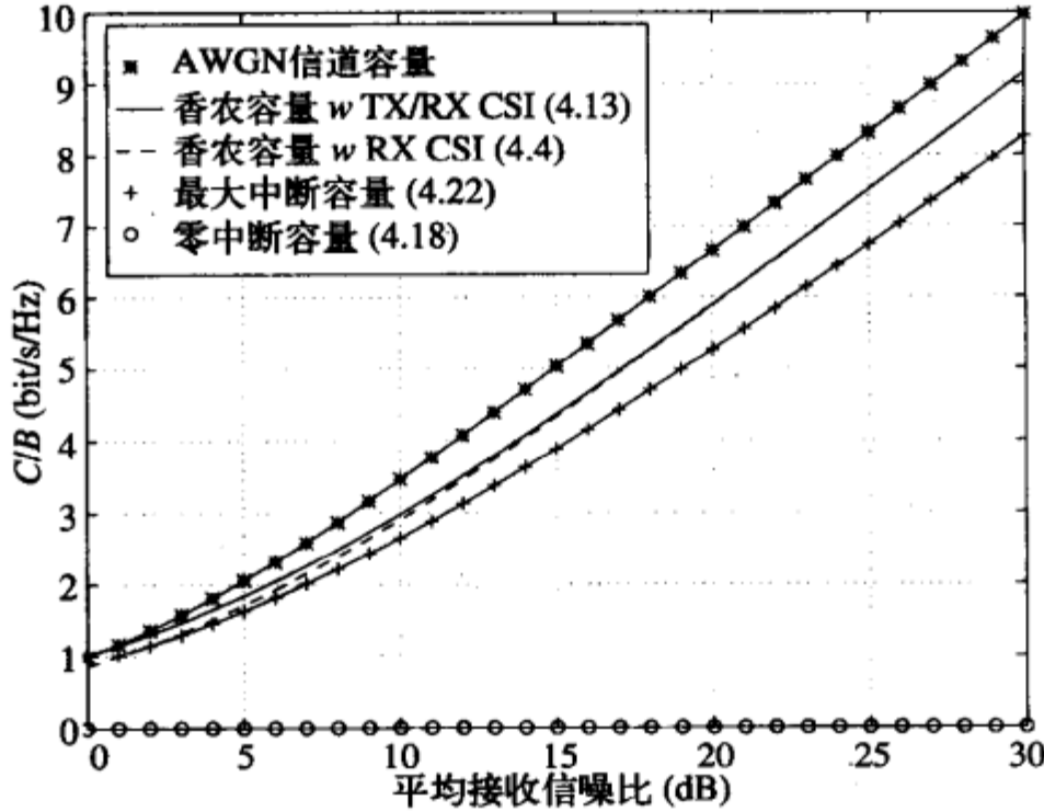
图4-7 瑞利衰落的容量
