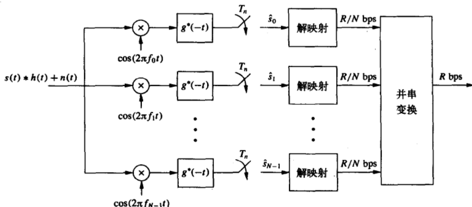
图12-4 重叠子载波系统的接收机
