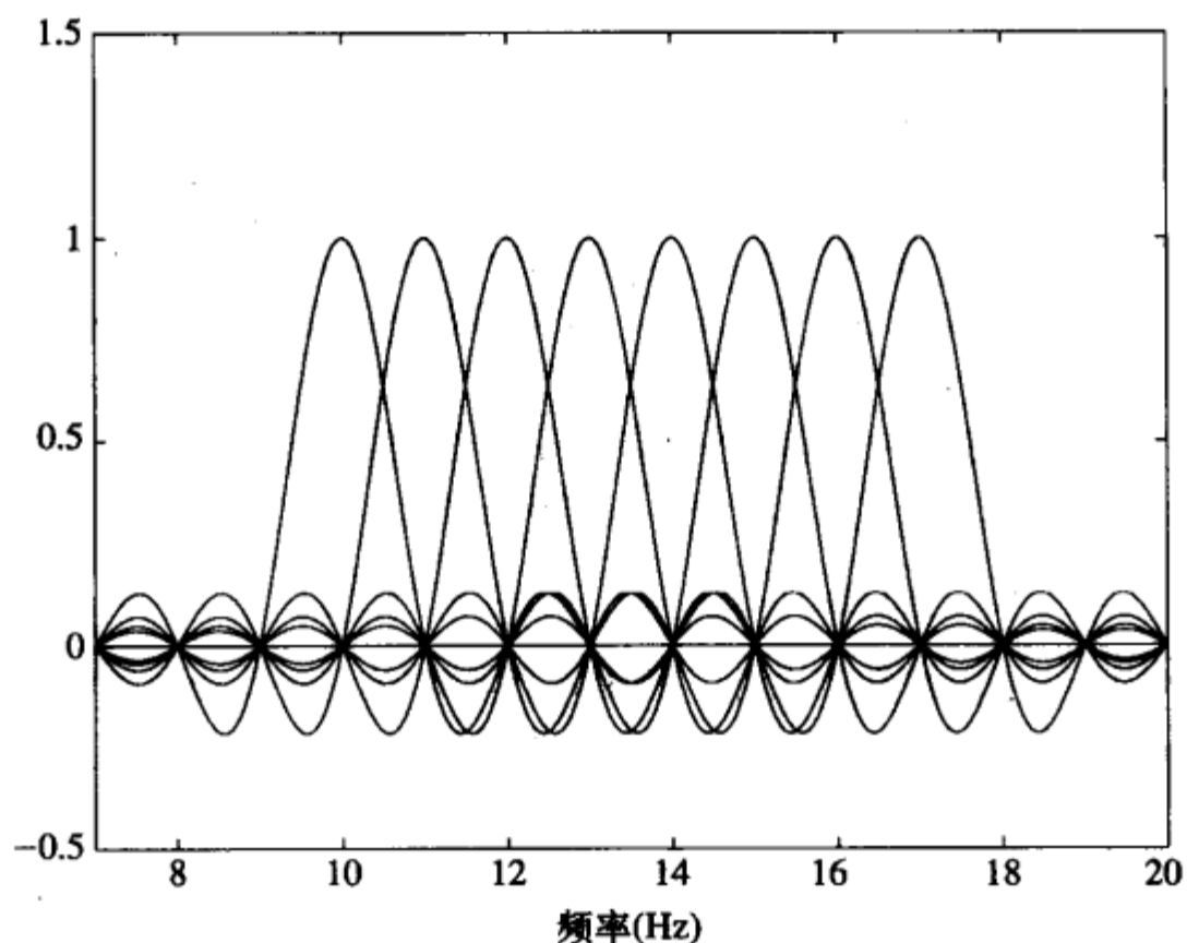
图12-12 重叠子载波的OFDM：矩形脉冲、 f_0 = 10\text{Hz} 、 \Delta f = 1\text{Hz}
