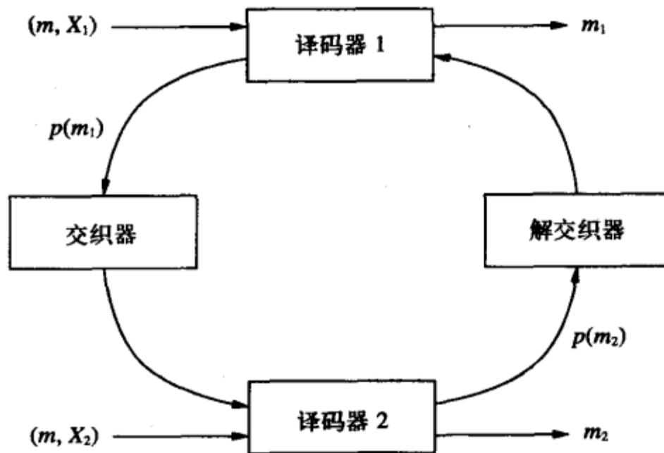
图8-15 Turbo码的译码器
