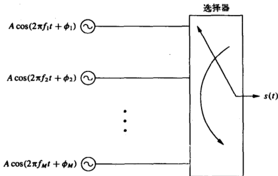
图5-22 频率调制器
