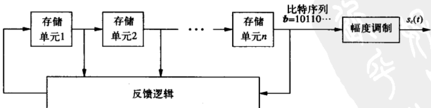
图13-6 扩频码的产生
