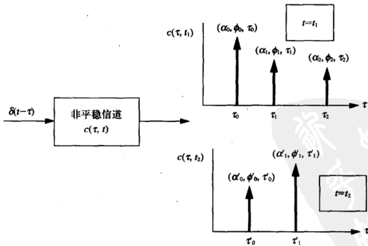
图3-3 非平稳信道的冲激响应
