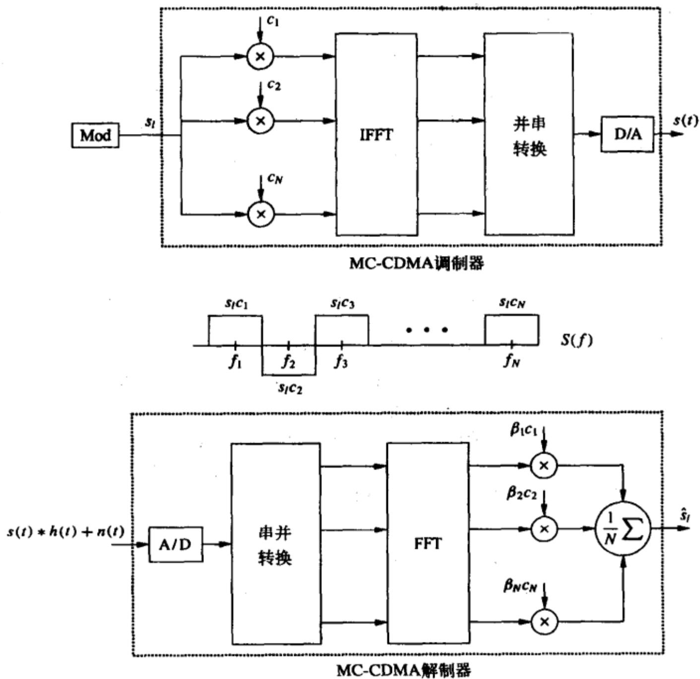
图13-17 多载波CDMA系统
