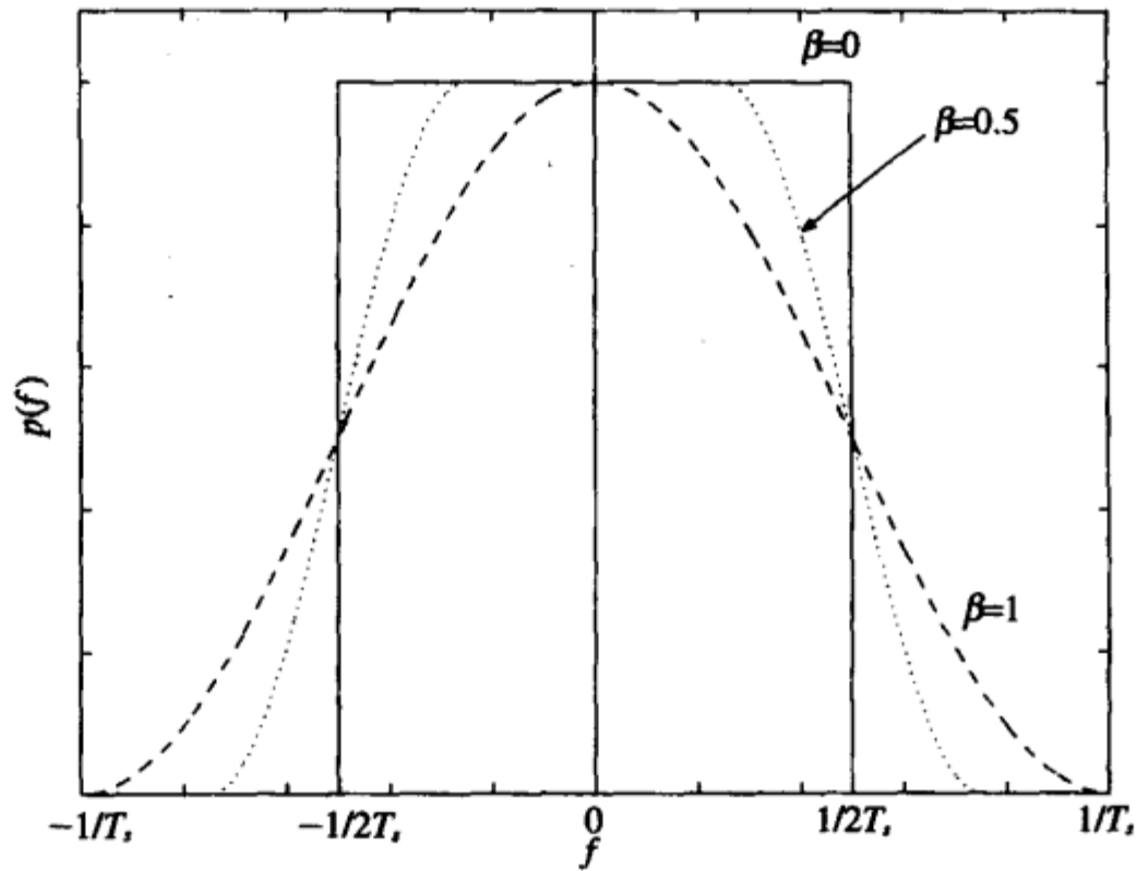
图5-26 升余弦脉冲的频域特性
