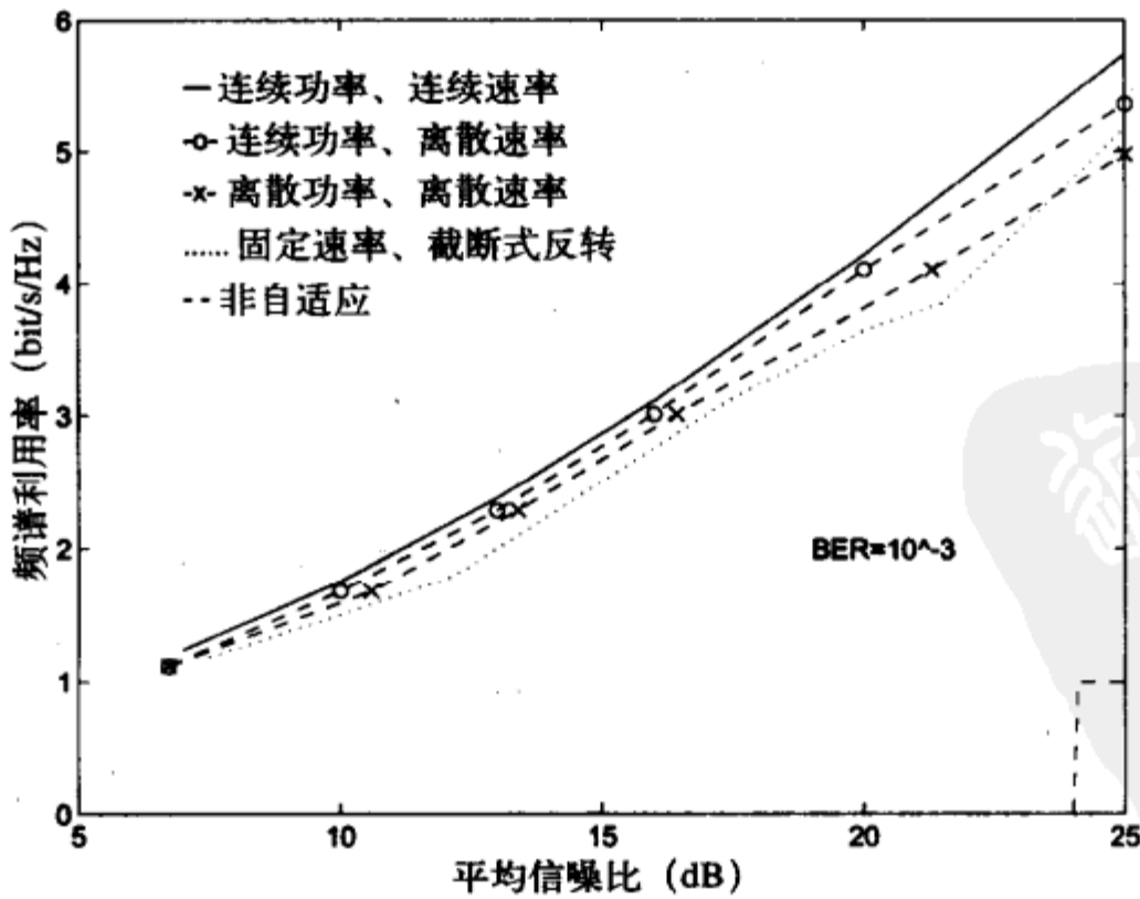
图9-8 瑞利衰落下的频谱利用率
