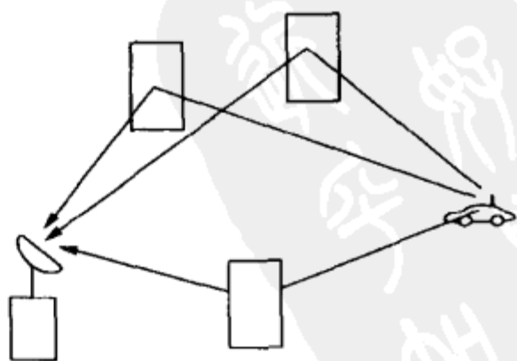
图3-16 散射点信道模型
