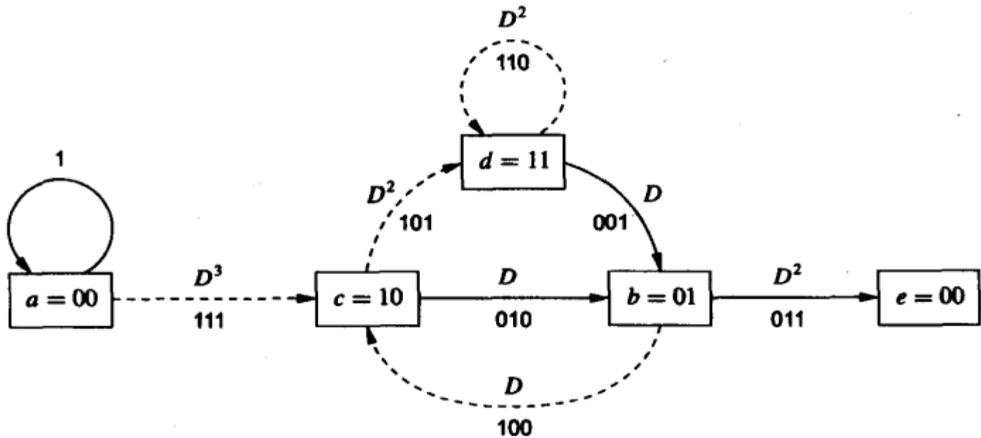
图8-11 状态图
