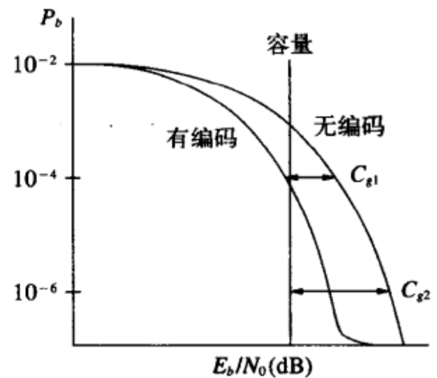
图8-1 AWGN信道下的编码增益
