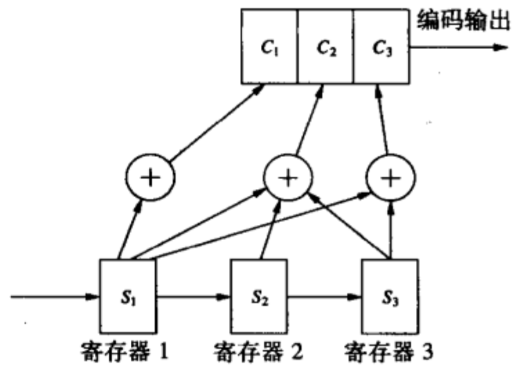
图8-6 卷积码编码器示例 ( n=3 、 k=1 、 K=3 )
