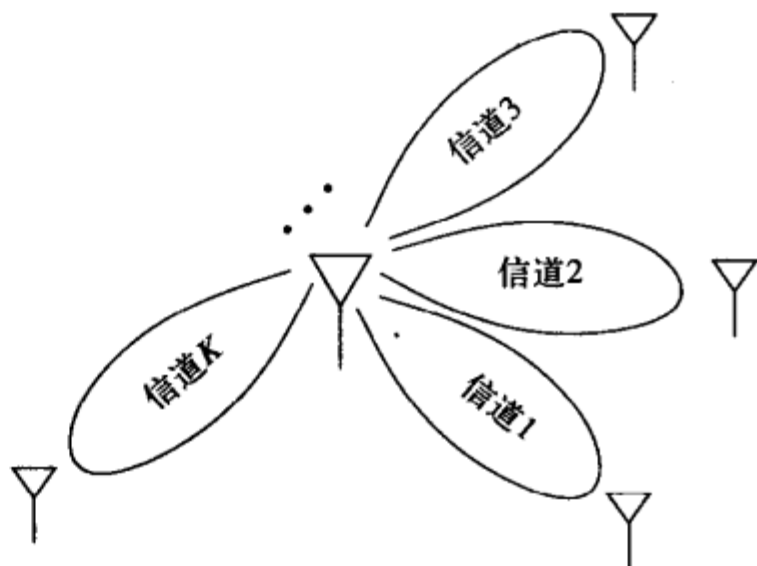
图14-5 空分多址
