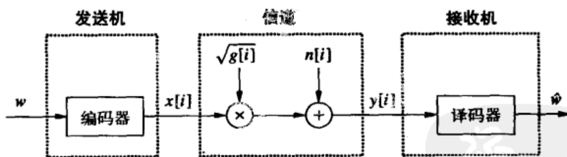
图4-1 平坦衰落信道及系统模型
