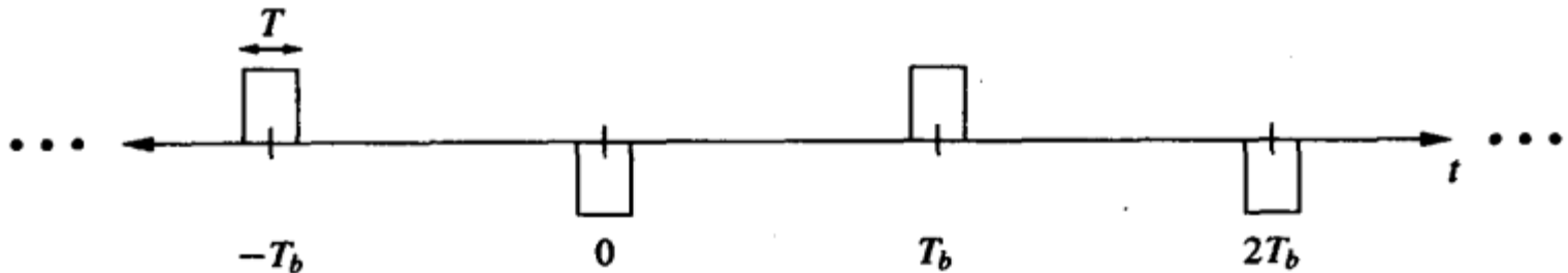
图11-6 习题11.16中UWB信号的形式
