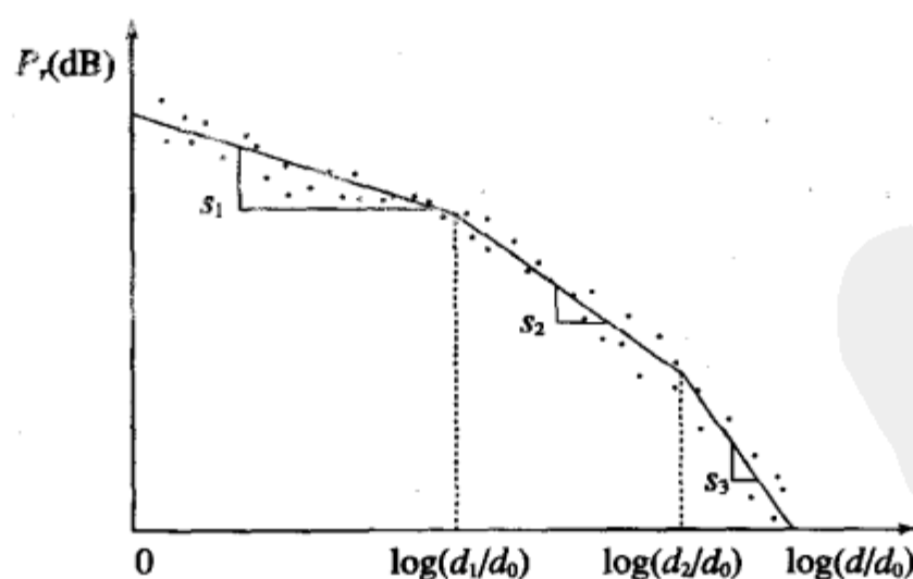
图2-9 路径损耗的折线模型
