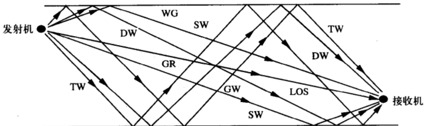
图2-6 十径模型的俯视图
