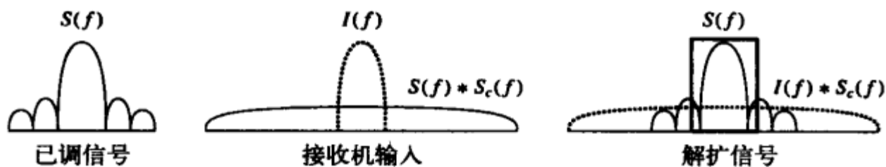
图13-2 直序扩频抗窄带干扰
