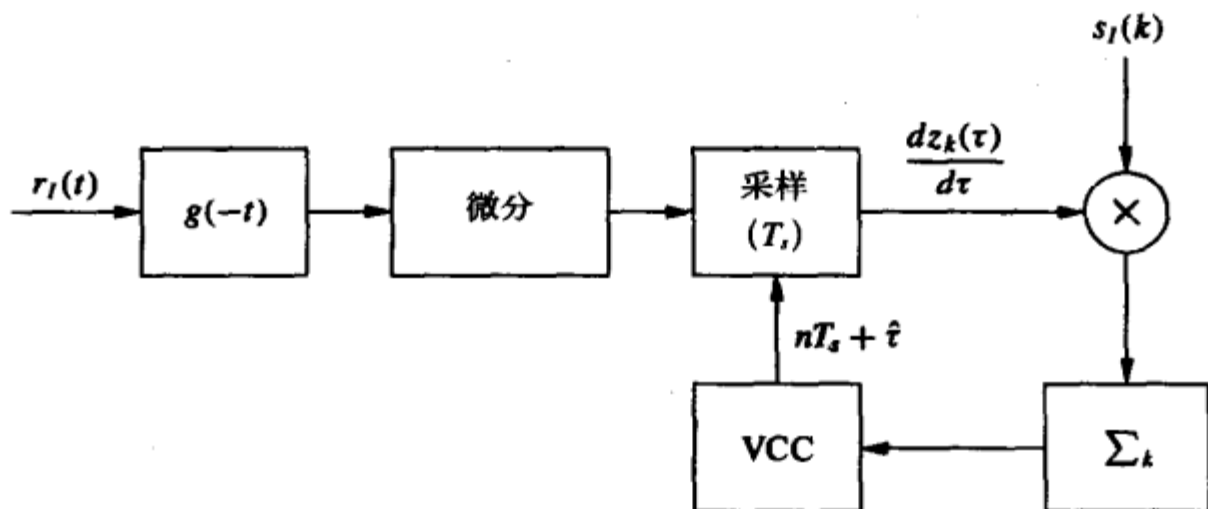
图5-30 非盲定时估计
