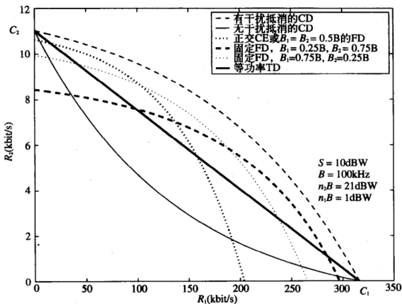
图14-11 两用户信噪比相差20dB时的容量域
