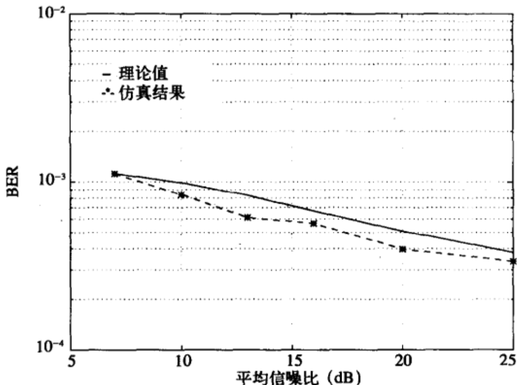
图9-10 瑞利衰落下的误比特率 (五个衰落区)
