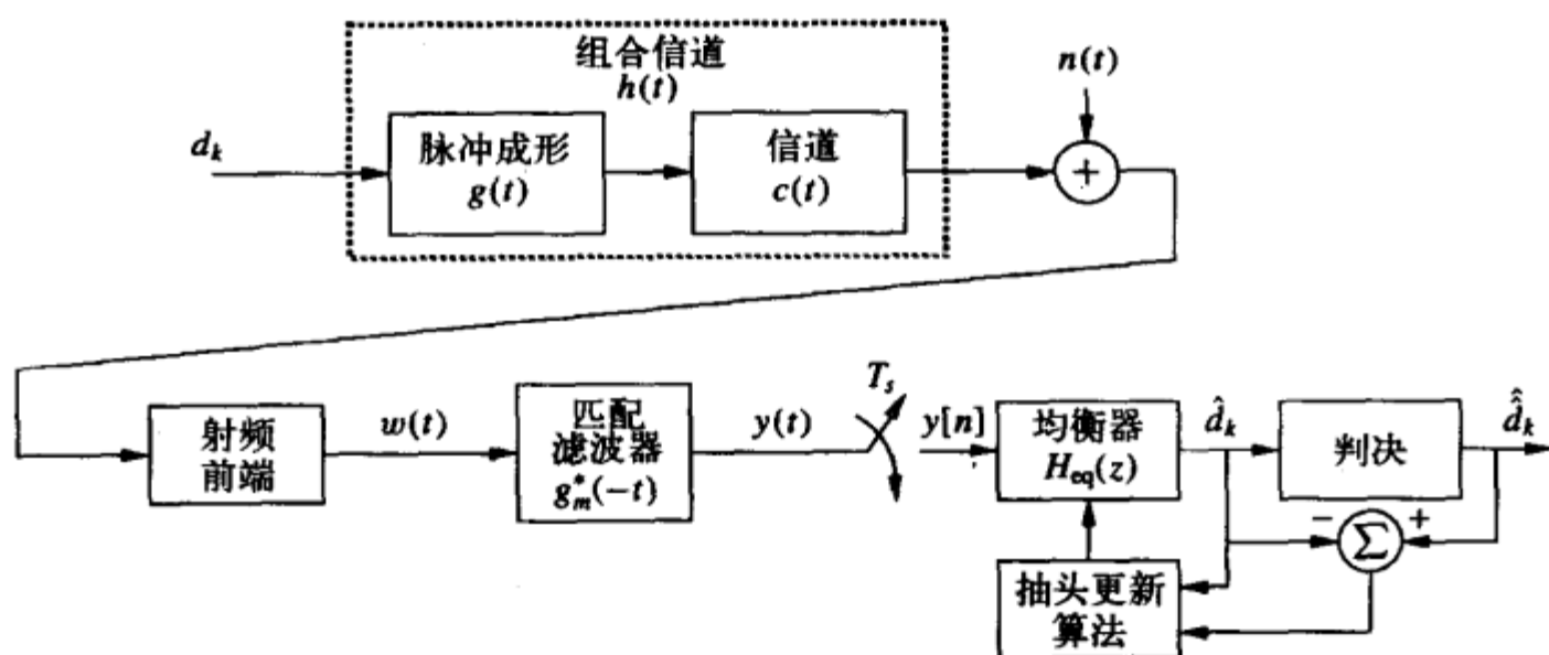
图11-3 端到端的等效基带系统
