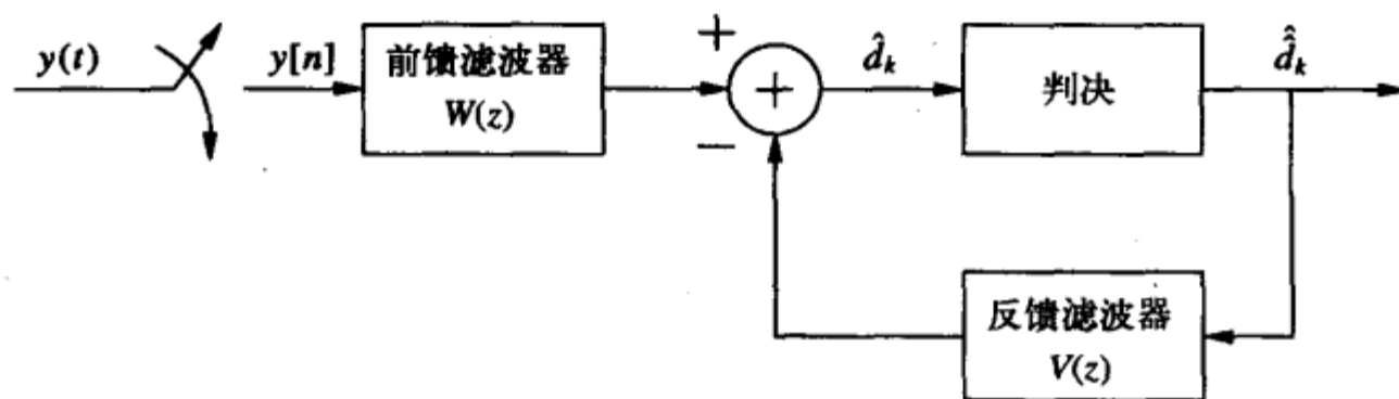
图11-5 判决反馈均衡器的结构
