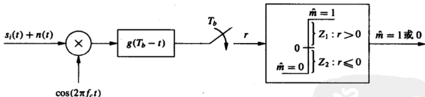
图5-17 BPSK的相干解调
