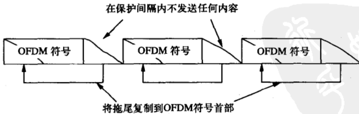
图12-8 用全零前缀产生循环信道
