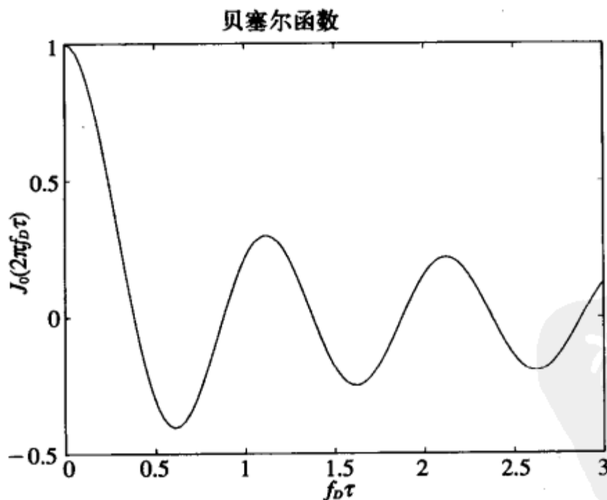
图3-5 以 f_D \tau 为自变量的贝塞尔函数
