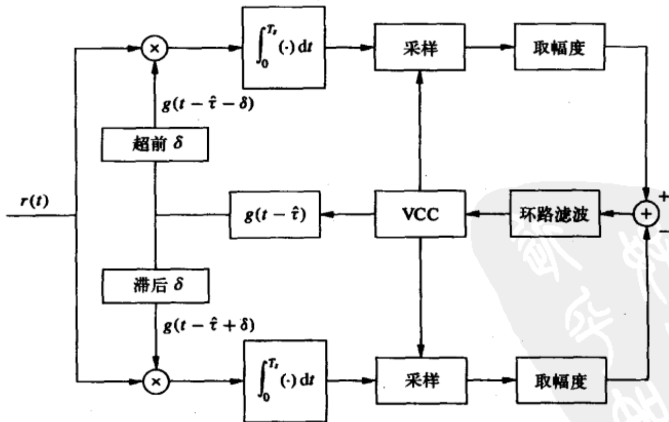
图5-31 超前一滞后门同步器
