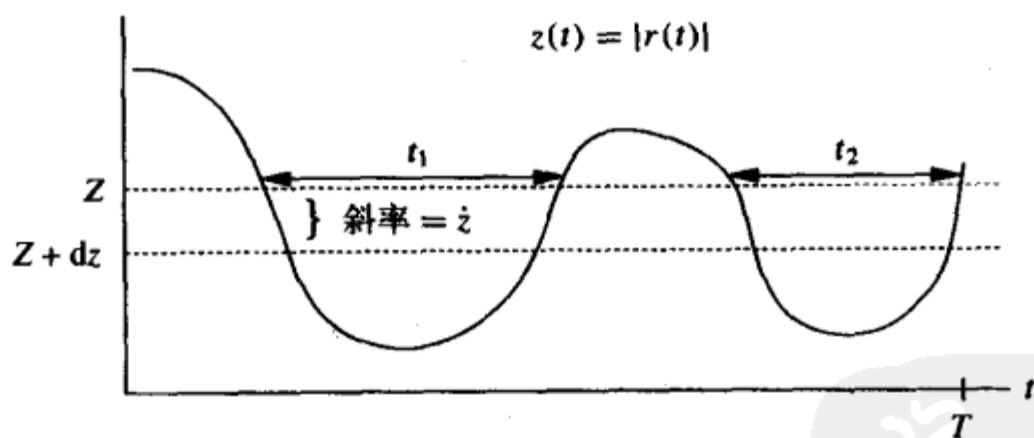
图3-10 衰落过程的电平通过率和衰落时长
