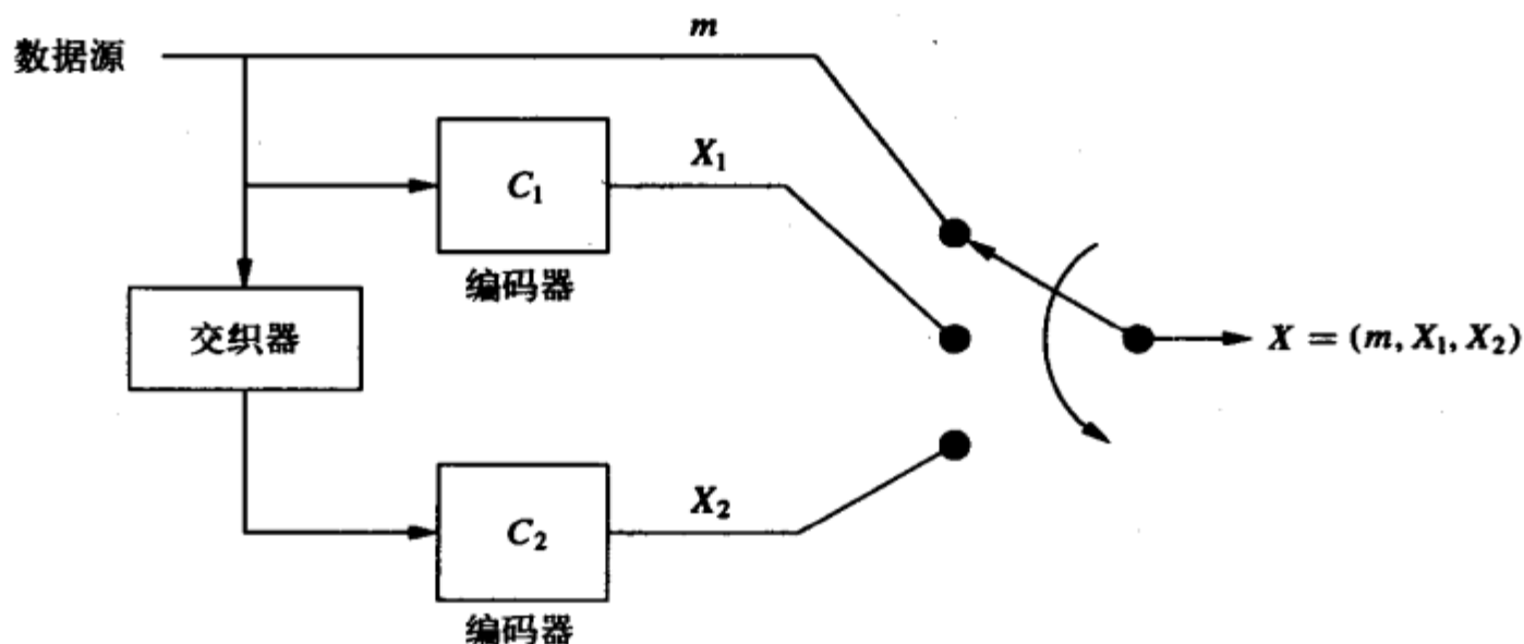
图8-14 并行级联码（Turbo码）的编码器
