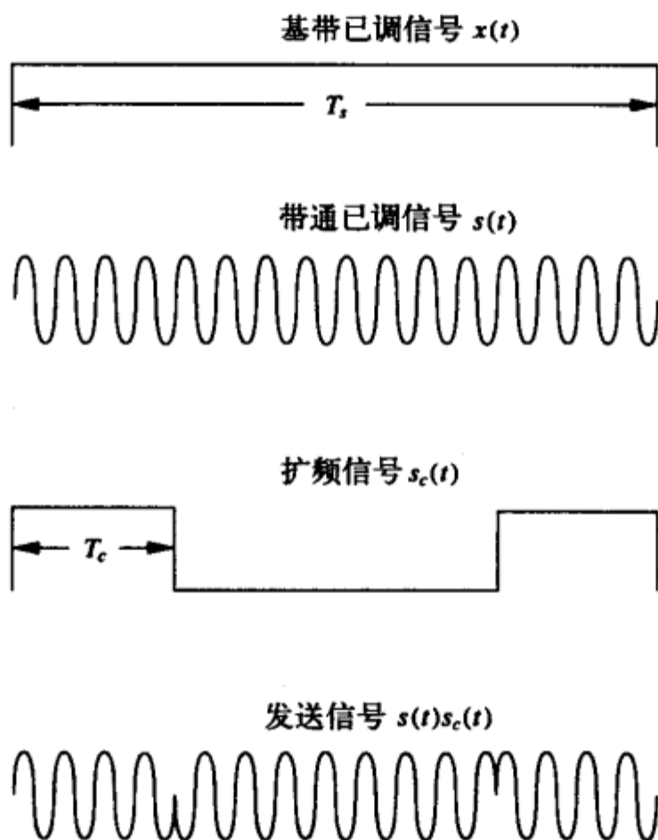
图13-1 扩频信号相乘
