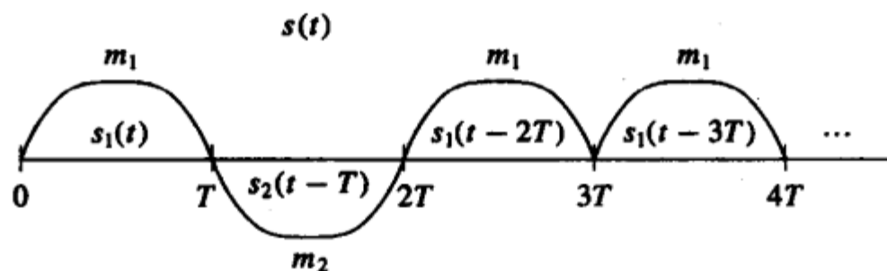
图5-2 消息序列对应的发送信号
