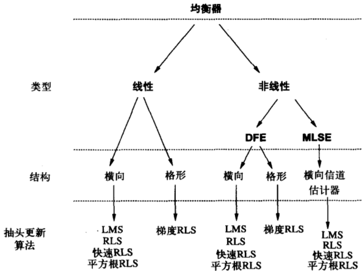
图11-2 均衡器的类型、结构和算法
