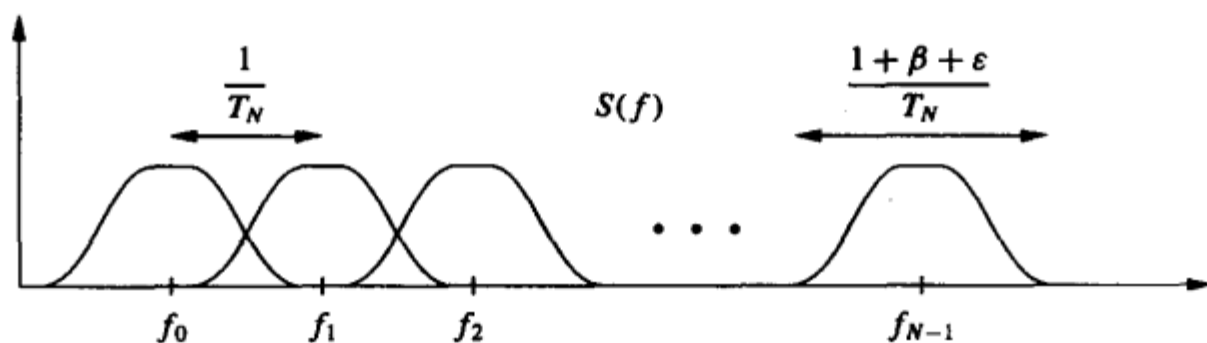
图12-3 子载波重叠的多个载波
