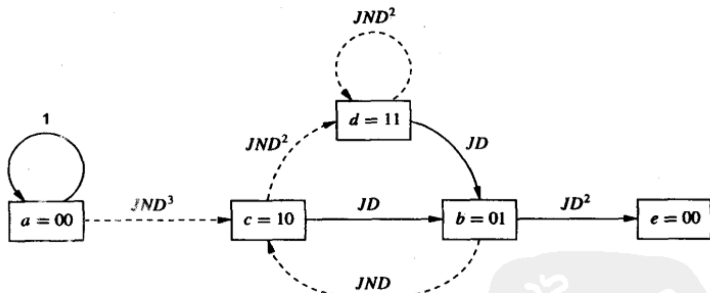
图8-12 扩展的状态图
