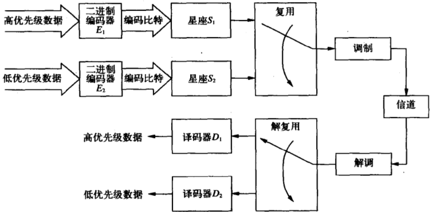
图8-22 时分复用的编码调制
