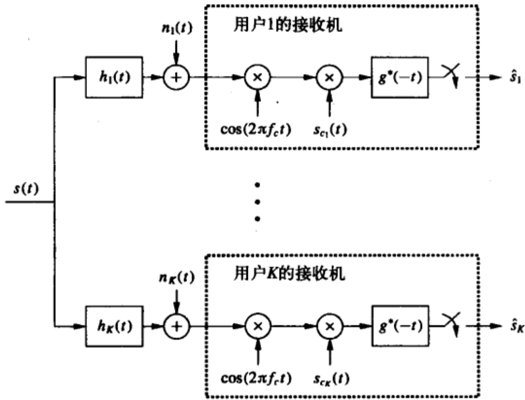
图13-14 下行信道及接收机
