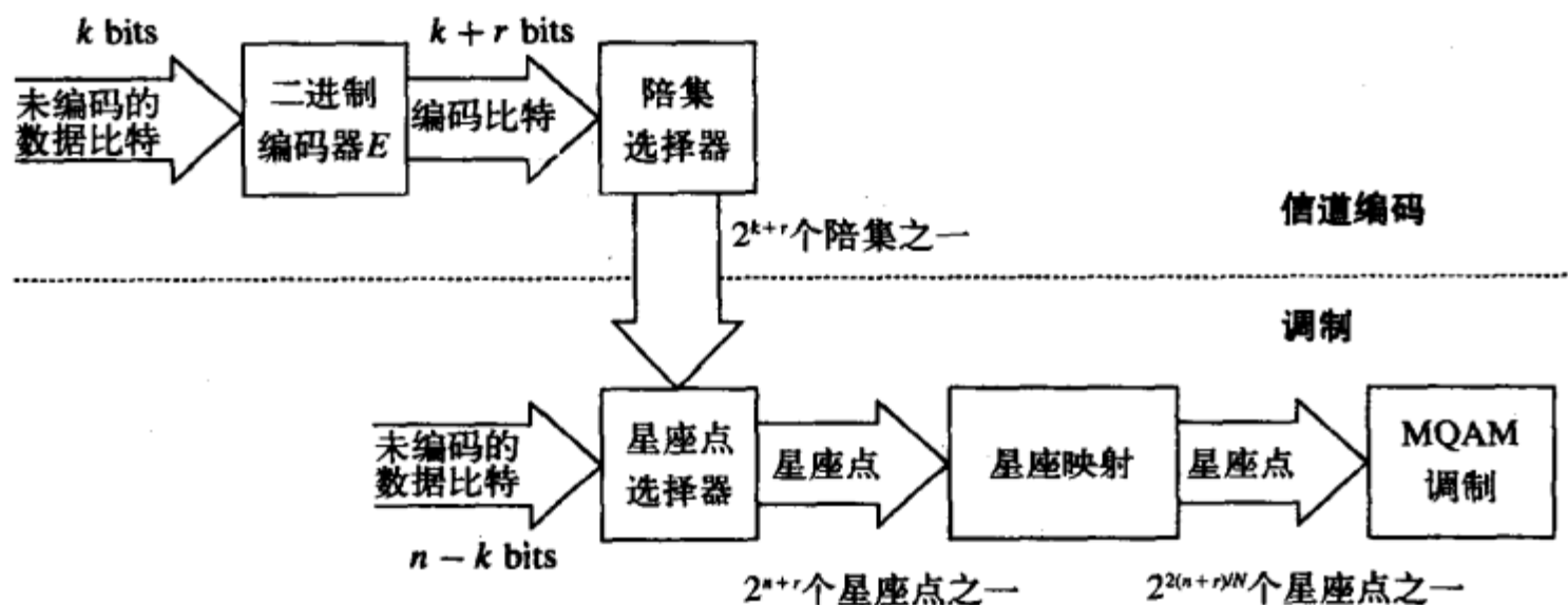
图8-17 编码调制的一般形式
