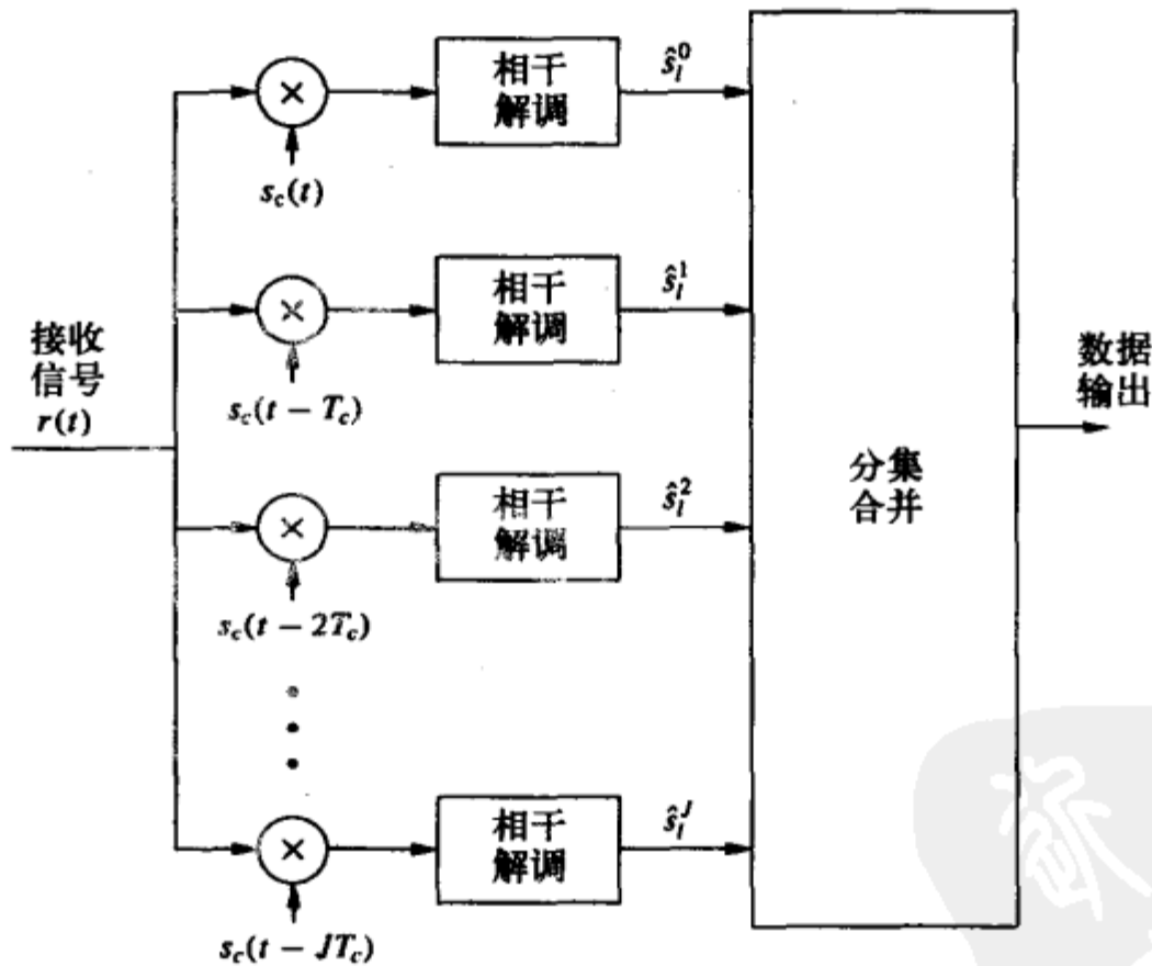
图13-10 RAKE接收机
