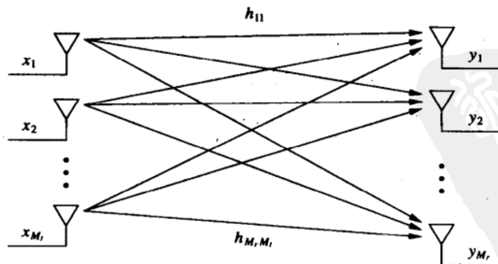
图10-1 MIMO系统
