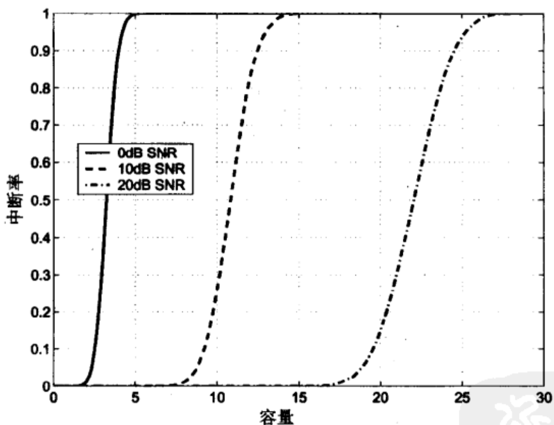
图10-6 4 \times 4 MIMO信道的中断率分布
