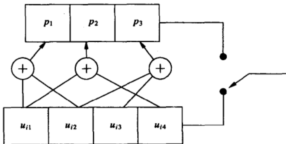
图8-2 二进制 (7,4) 码的实现
