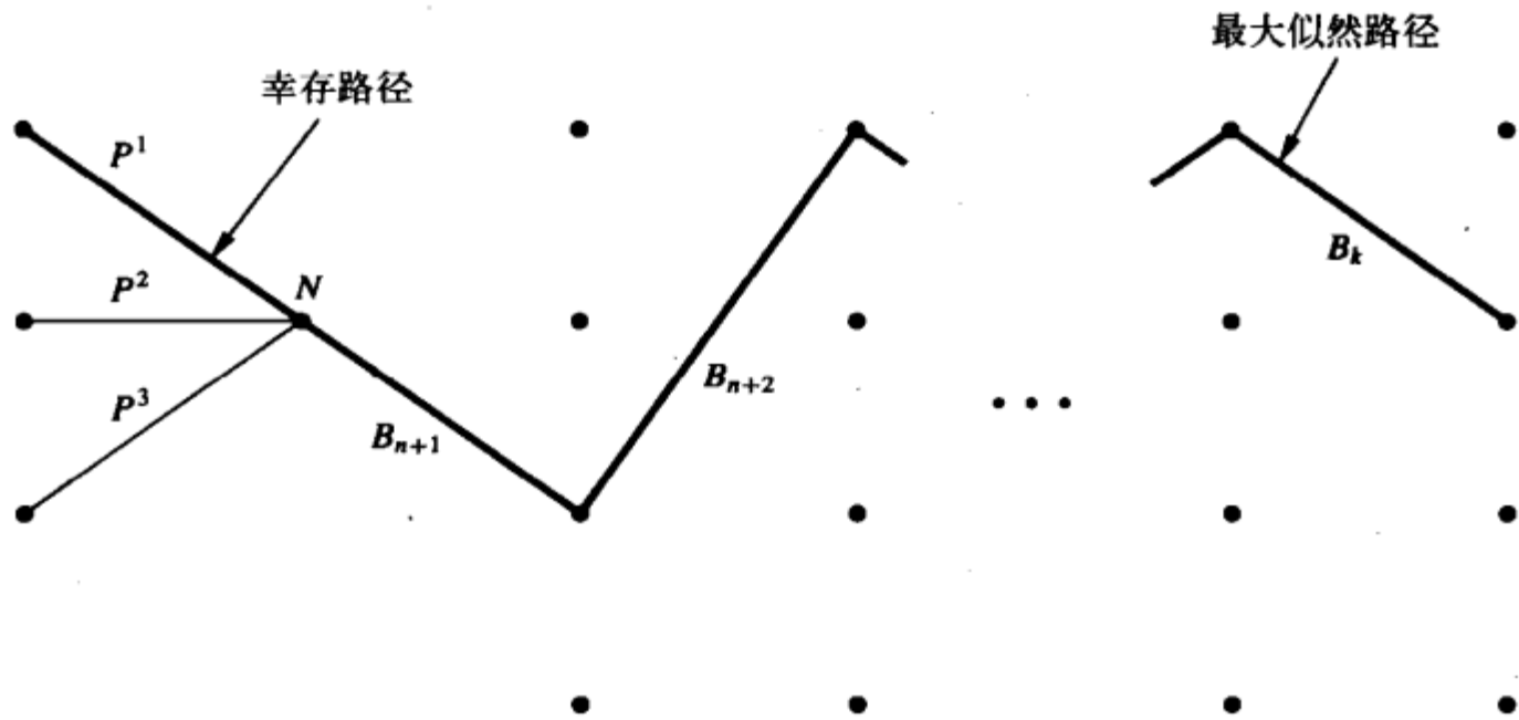
图8-8 最大似然路径上的部分路径度量
