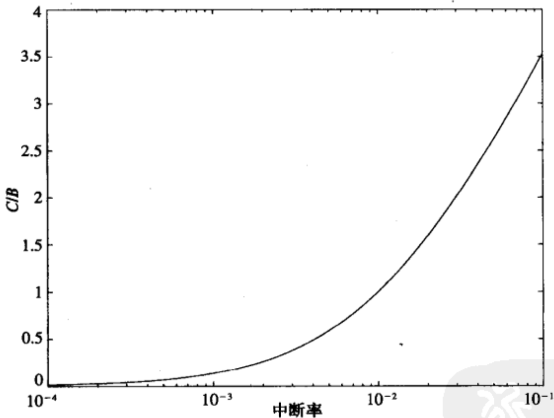
图4-2 归一化容量 ( C/B ) 与中断率的关系
