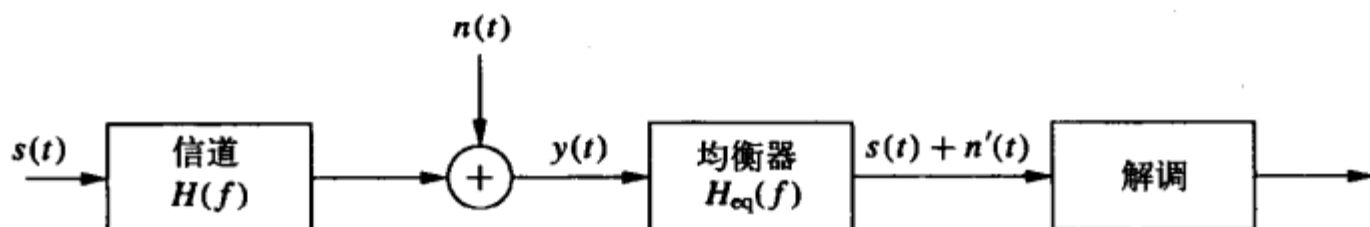
图11-1 通过模拟均衡器说明噪声增强
