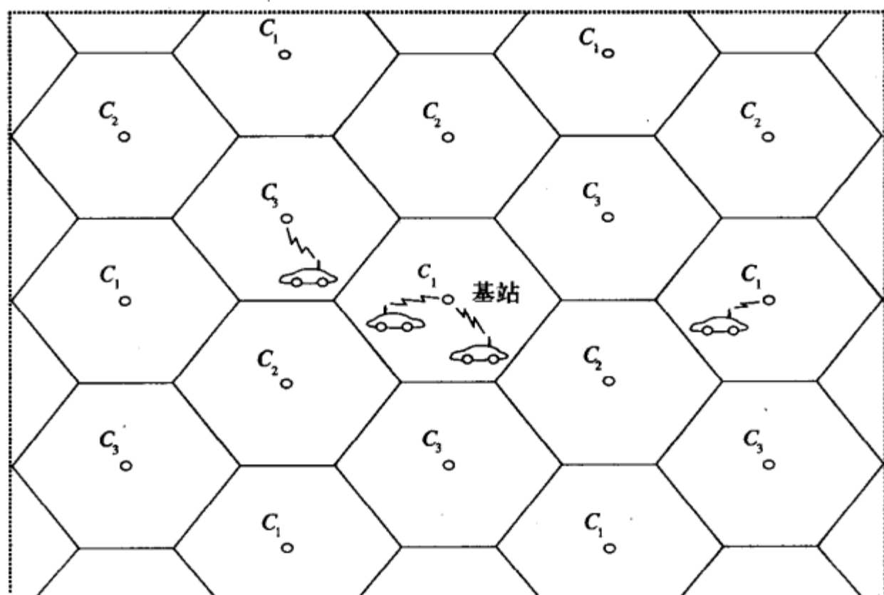
图1-1 蜂窝系统
