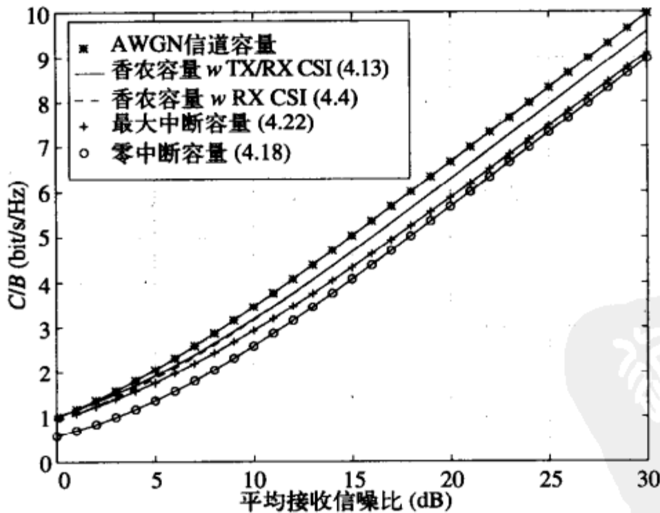
图4-8 Nakagami衰落 ( m=2 ) 的容量
