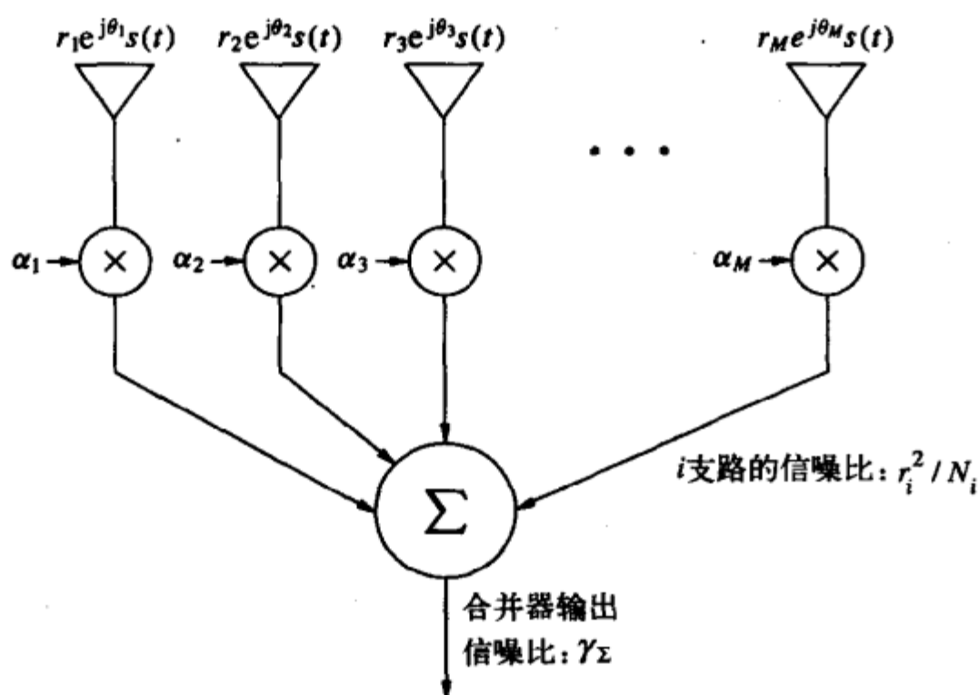
图7-1 线性合并器
