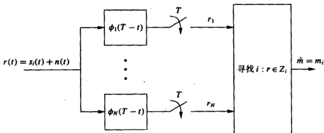
图5-7 匹配滤波接收机结构
