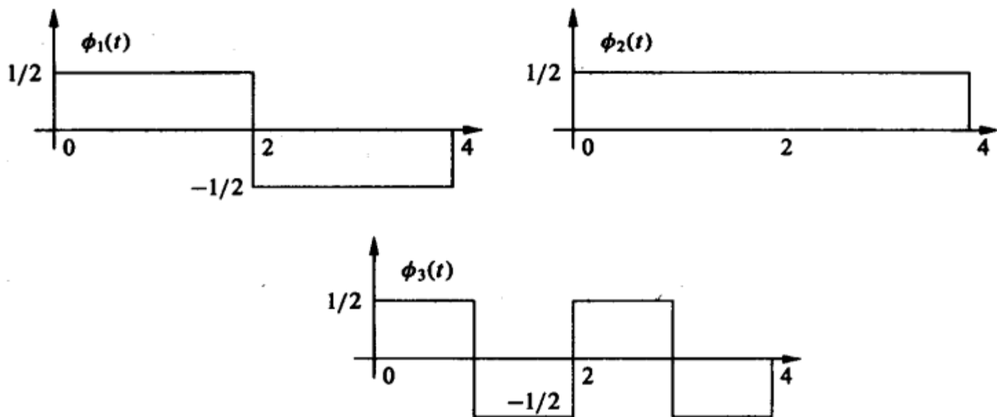
图5-32 题5.4的信号波形
