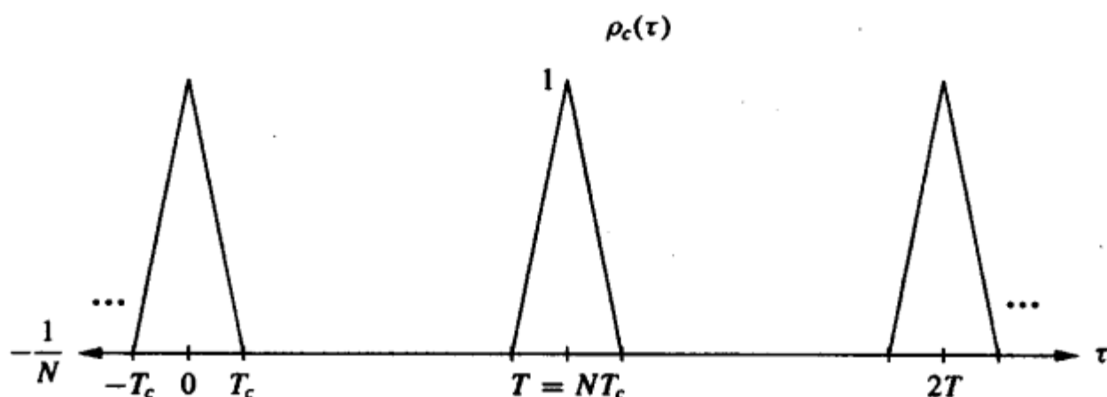
图13-8 周期为 T=NT_c 的自相关函数
