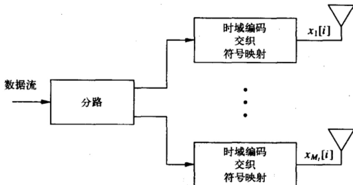
图10-10 并行编码的空分复用：V-BLAST
