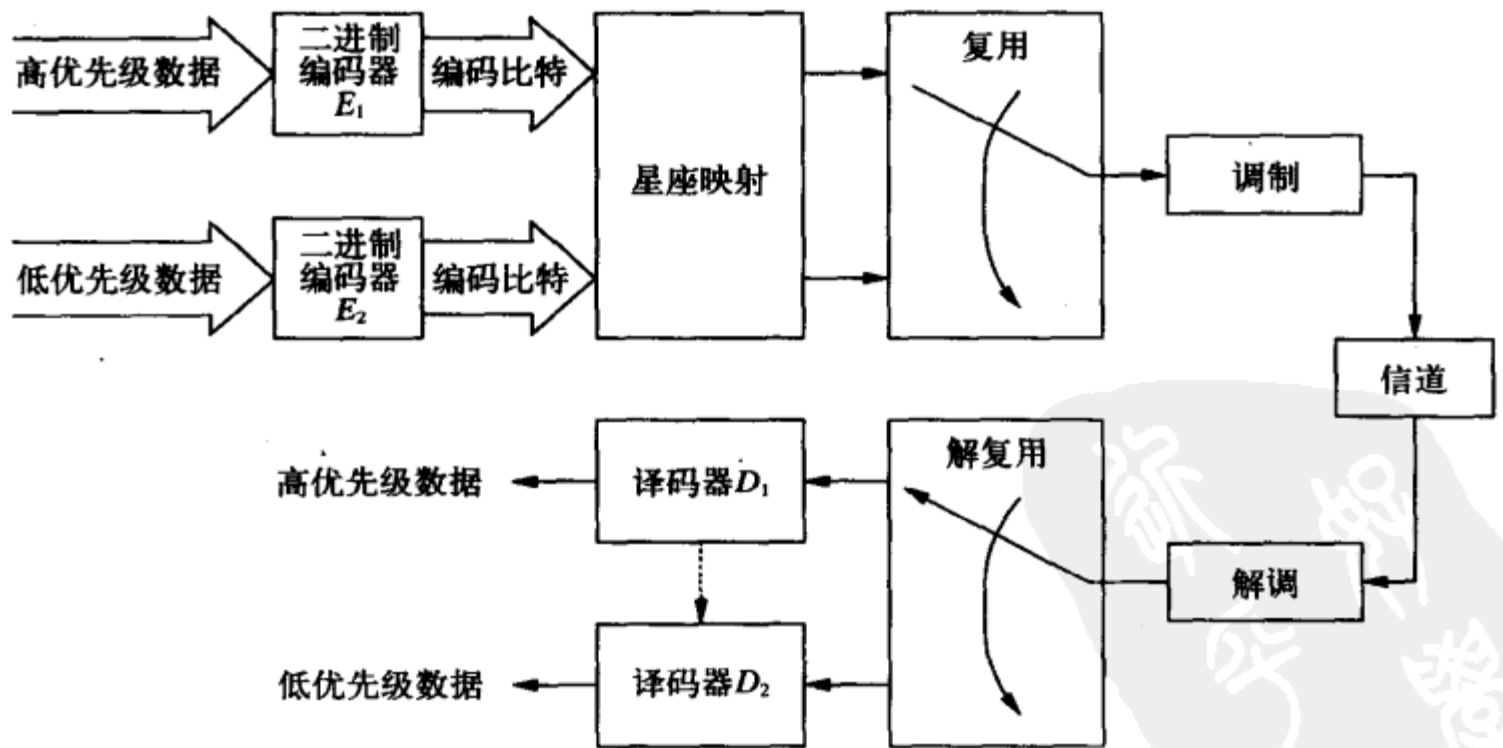
图8-23 信号星座的联合最优化
