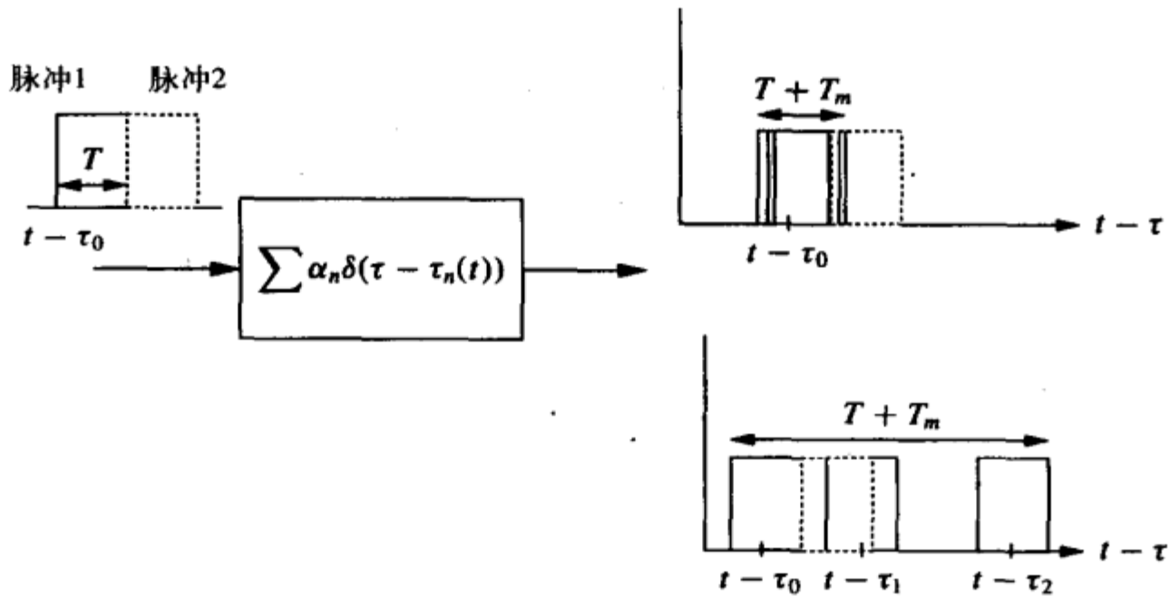
图3-11 多径的分辨性
