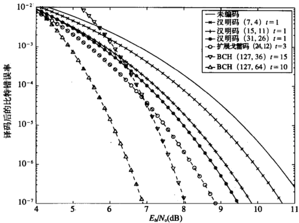
图8-4 不同BCH码的比特错误率
