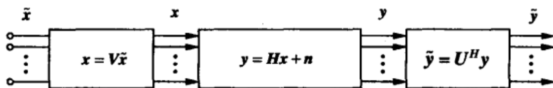
图10-2 发送预编码和接收成形
