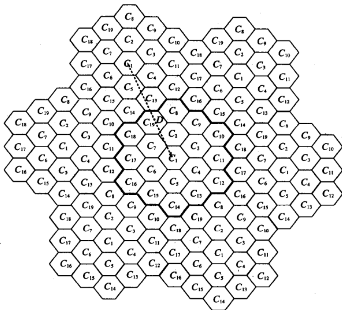
图15-7 正六边形小区的小区簇
