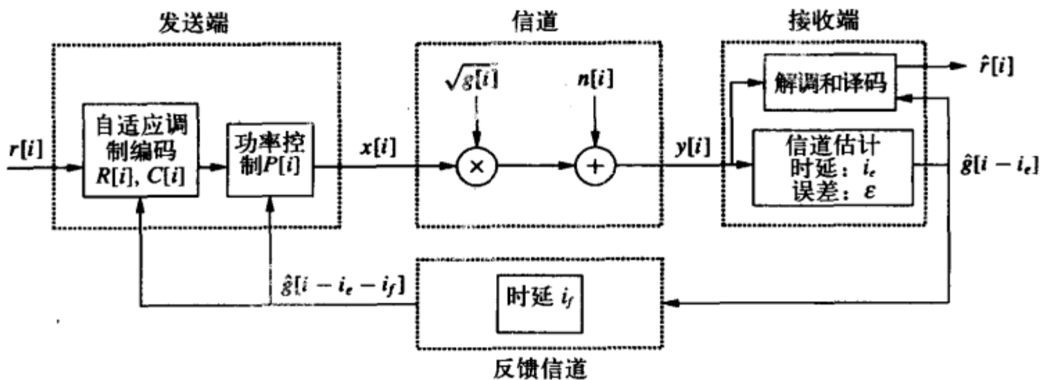
图9-1 系统模型
