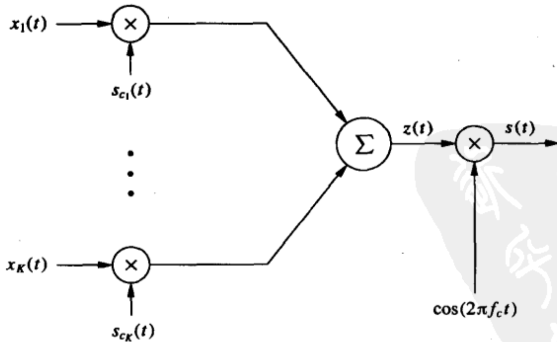
图13-13 下行链路的发送端
