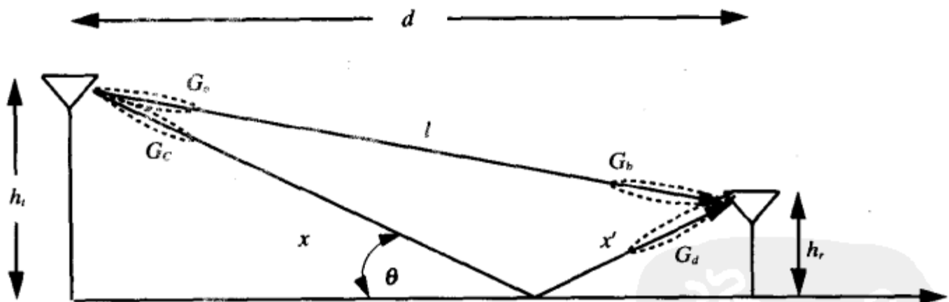
图2-4 两径模型
