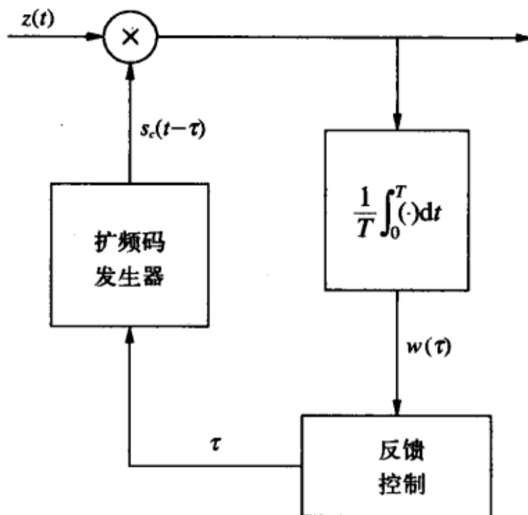
图13-9 DSSS中的同步环路
