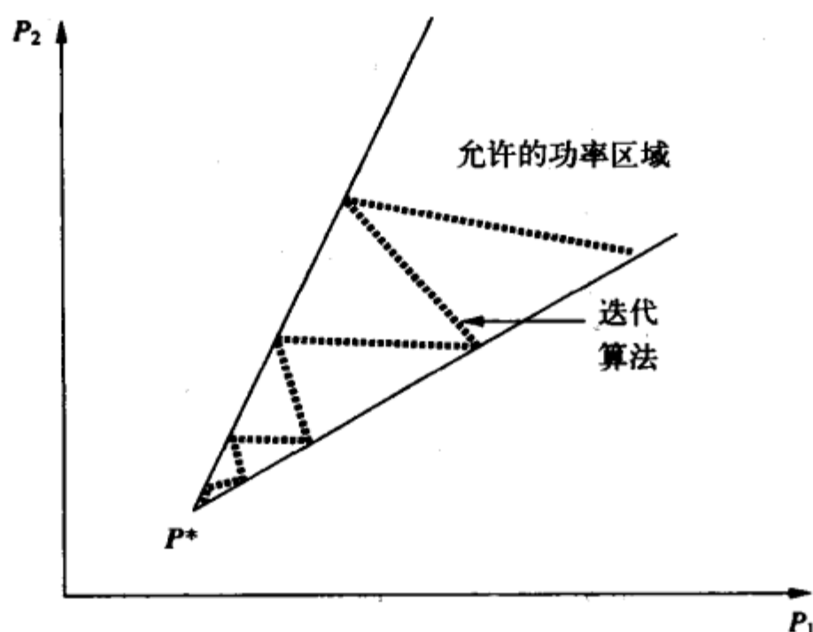
图14-8 迭代Foschini-Miljanic算法
