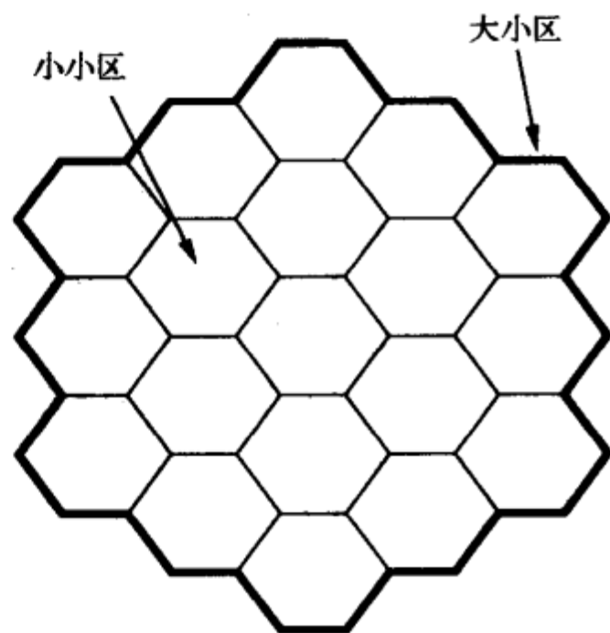
图15-2 容量随着小区的缩小而增加
