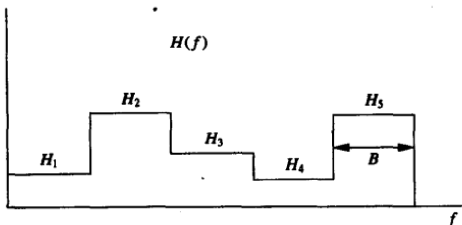
图4-10 分块频率选择性衰落
