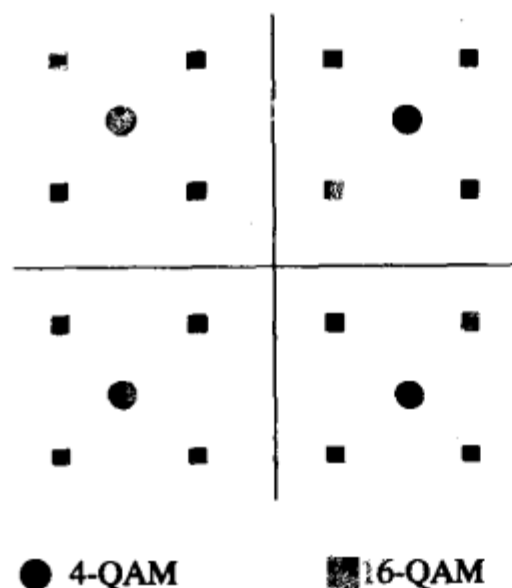
图5-18 4-QAM和16-QAM星座
