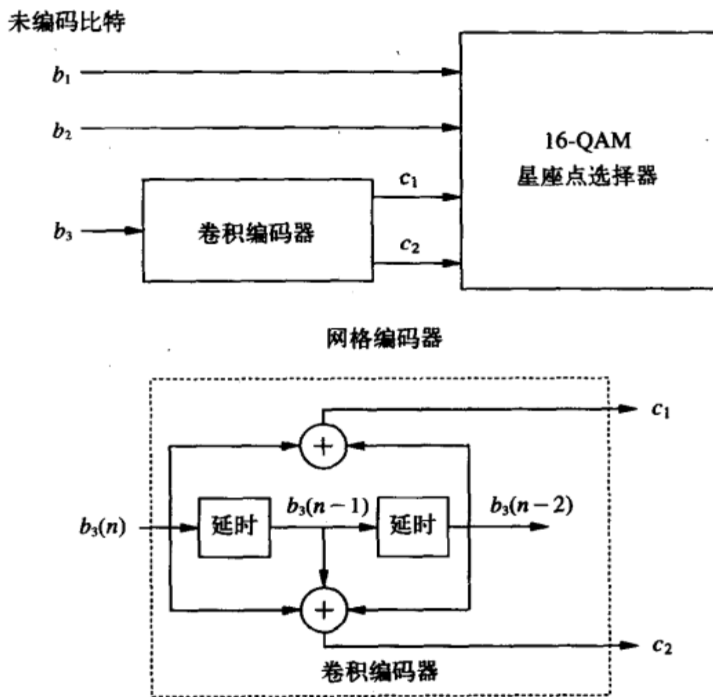
图8-25 题8.16中的16-QAM网格编码器
