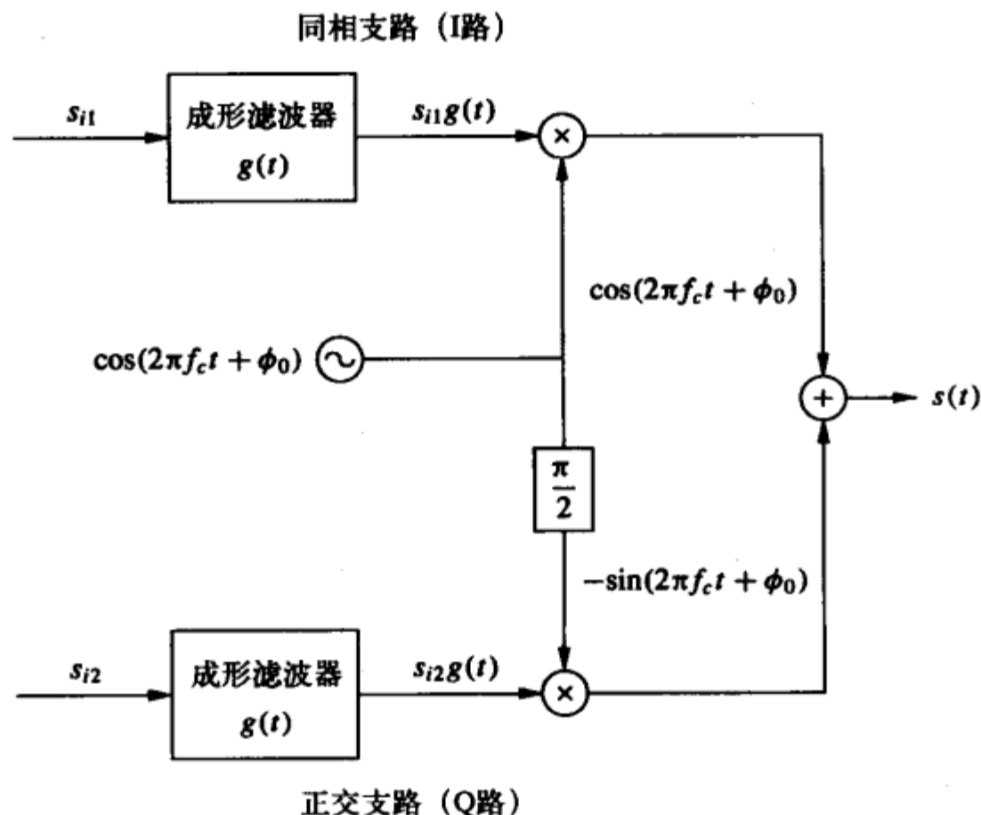
图5-10 幅度/相位调制器
