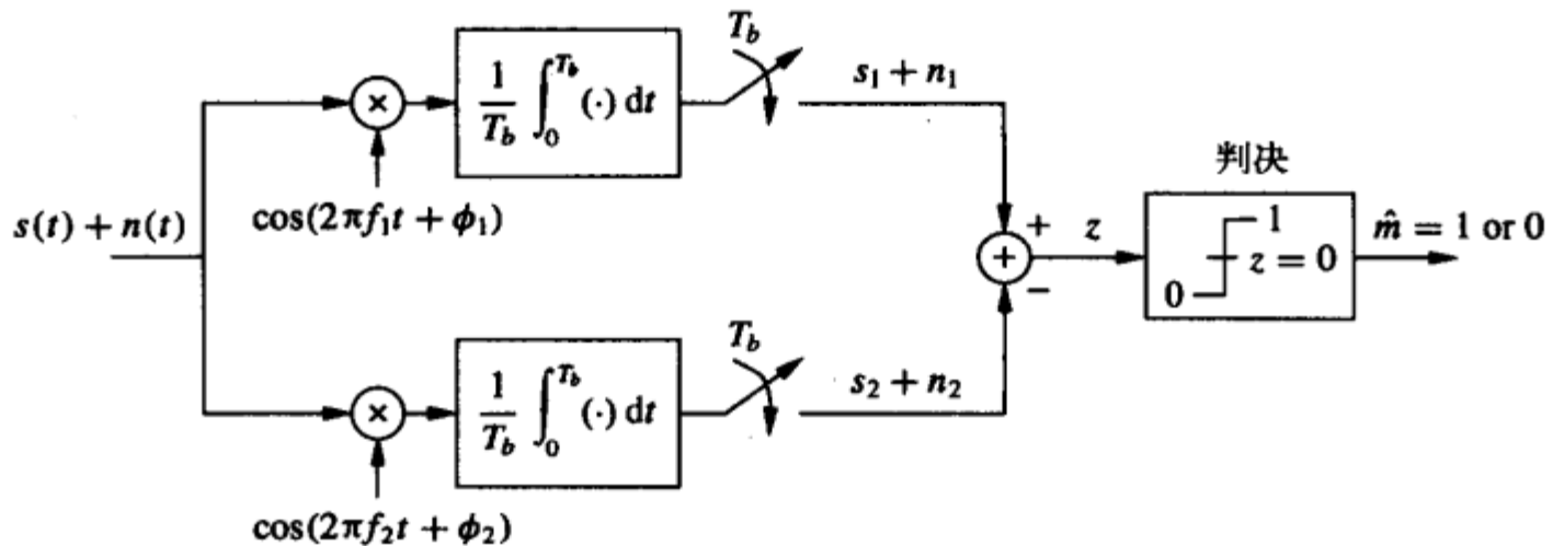
图5-24 2FSK解调器
