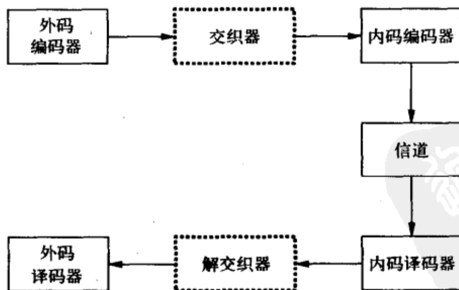
图8-13 级联码
