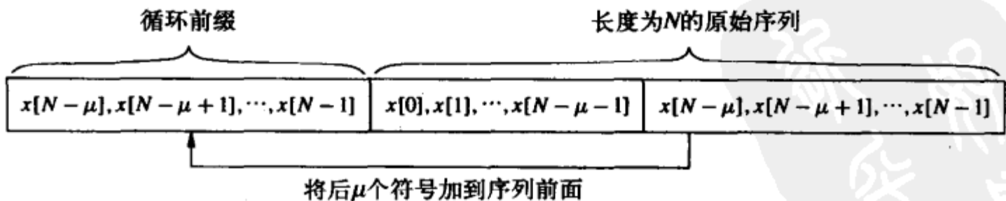
图12-5 长度为 \mu 的循环前缀
