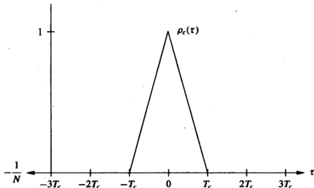
图13-7 最大线性码的自相关函数 ( N=T/T_c )
