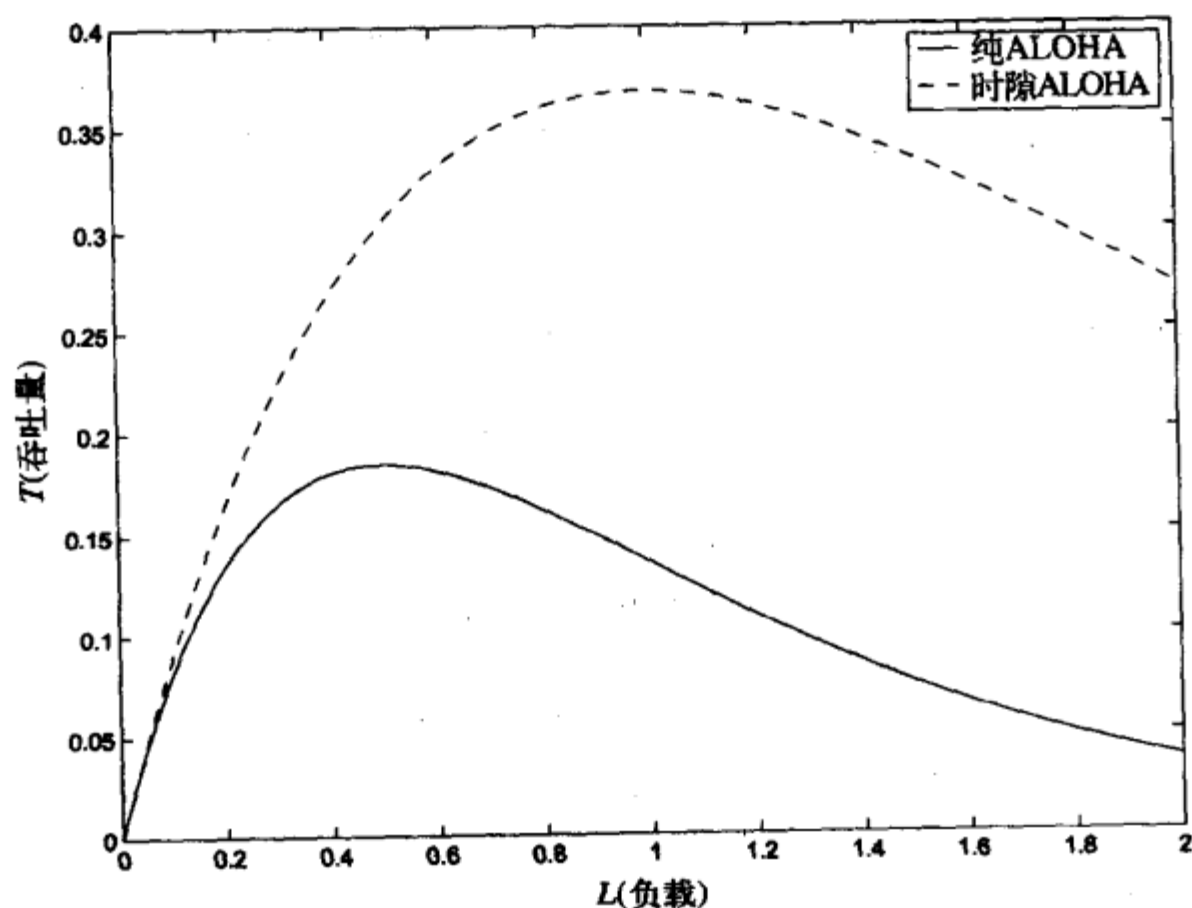
图14-6 纯ALOHA和时隙ALOHA的吞吐量
