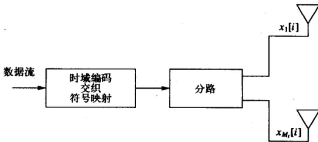
图10-9 串行编码的空分复用
