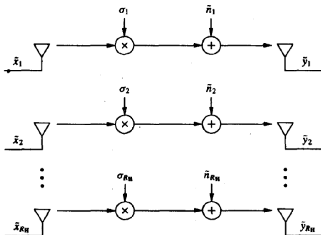
图10-3 MIMO信道的并行分解
