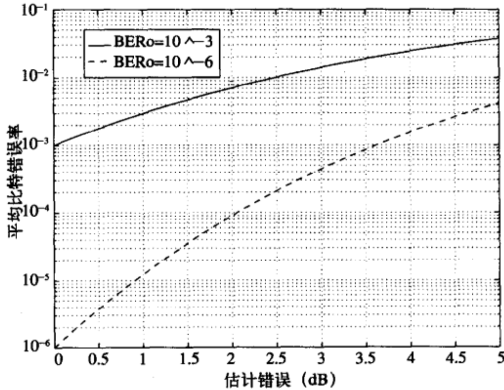
图9-11 估计错误给BER带来的影响
