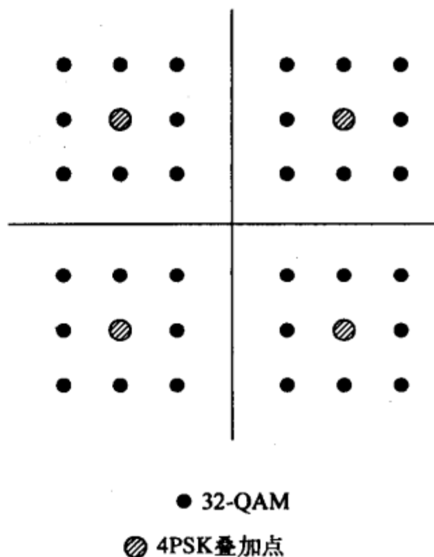
图14-9 嵌入4PSK的32-QAM
