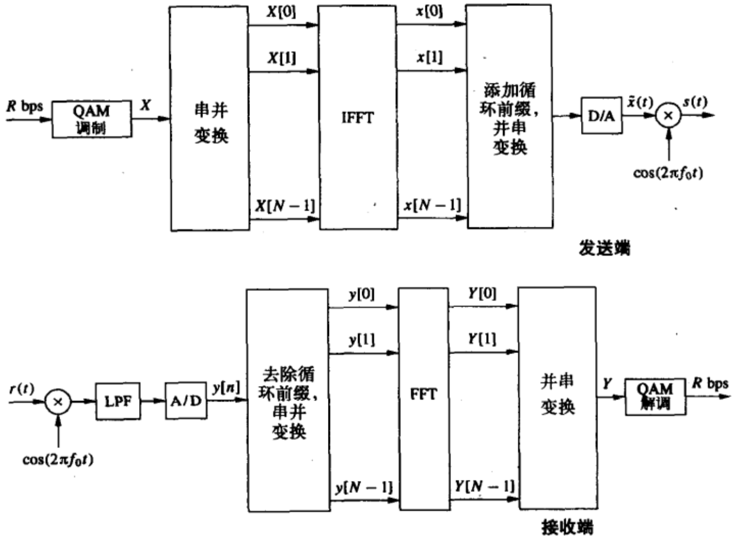
图12-7 用IFFT/FFT实现OFDM
