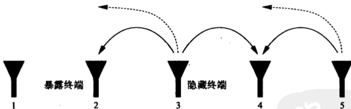
图14-7 隐藏终端和暴露终端
