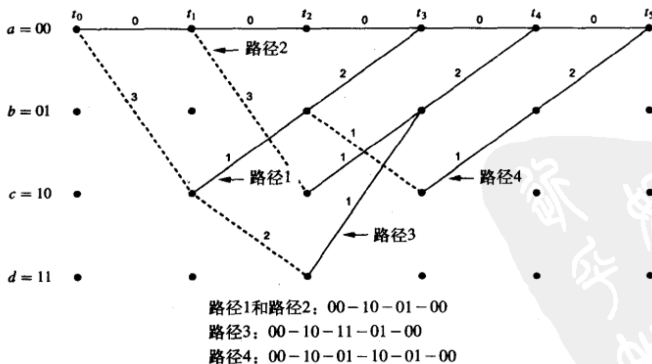
图8-10 与全零路径的距离
