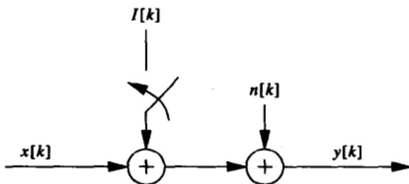
图4-13 题4.8中的干扰信道
