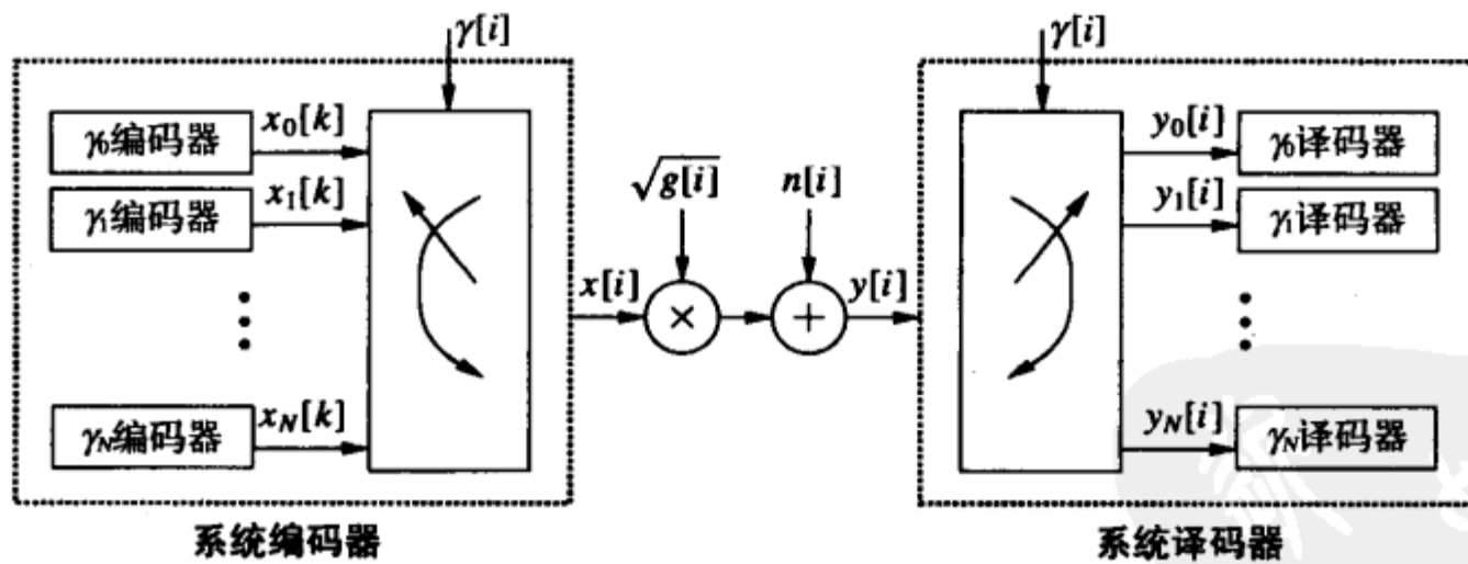
图4-4 编译码多路复用
