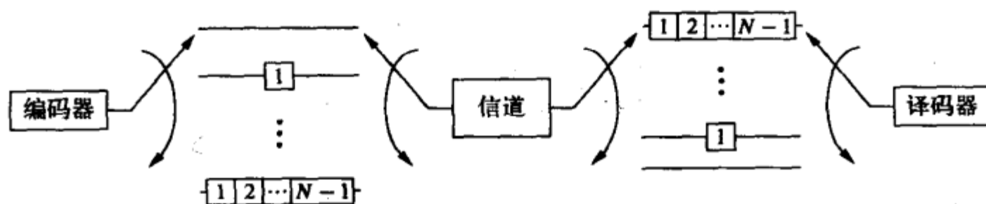
图8-20 卷积交织
