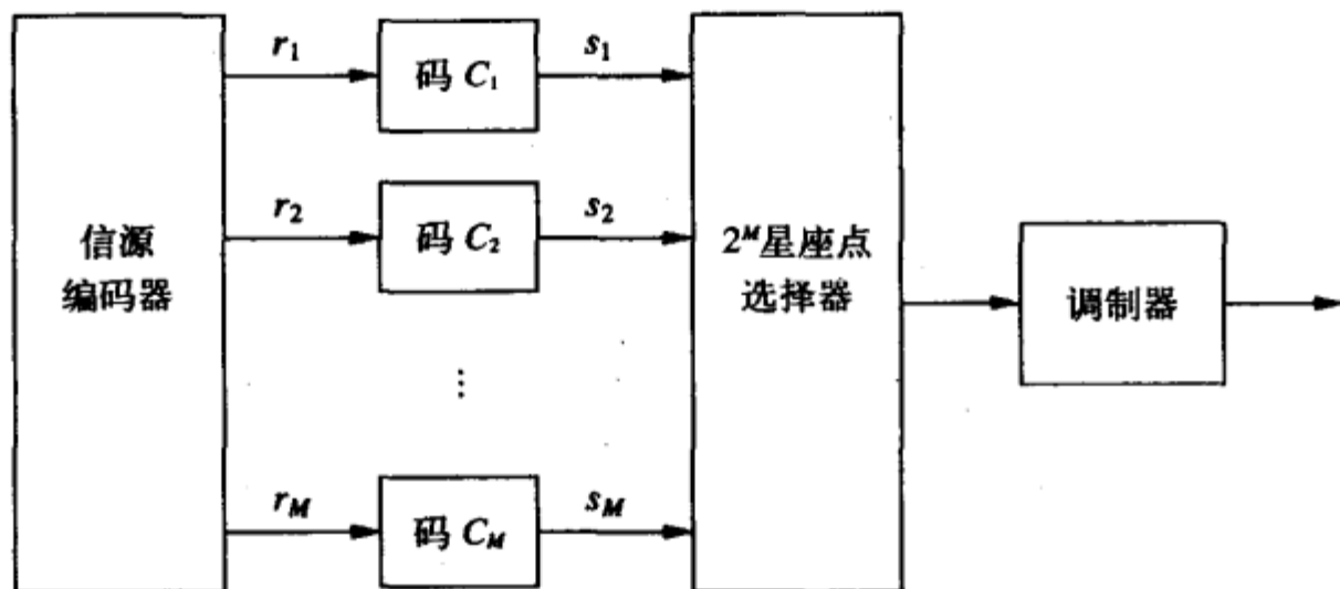
图8-21 多电平编码
