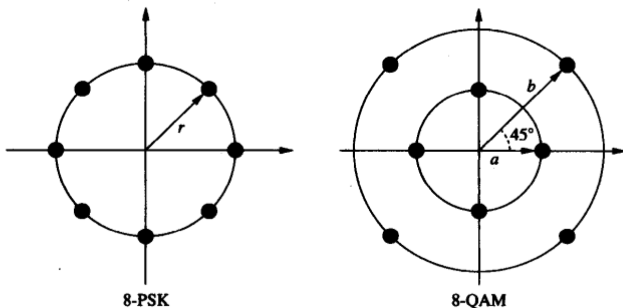
图5-34 题5.17的八进制星座图
