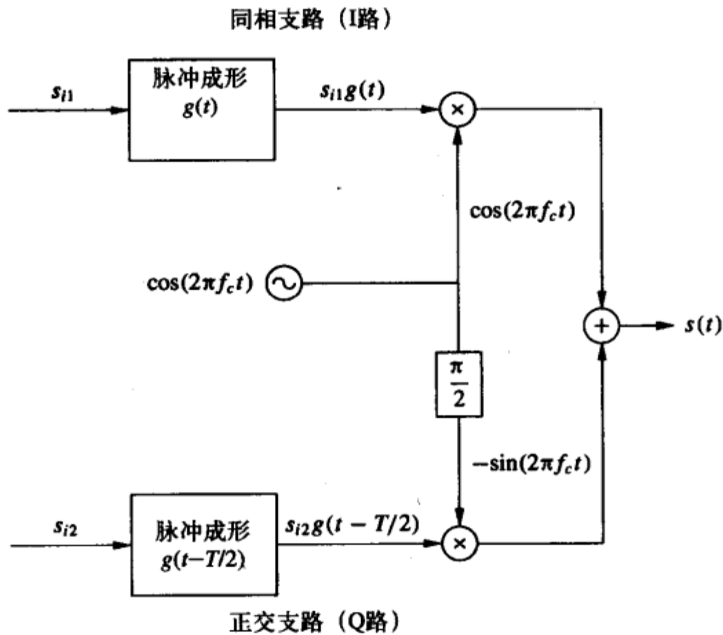
图5-21 带正交偏移的调制器
