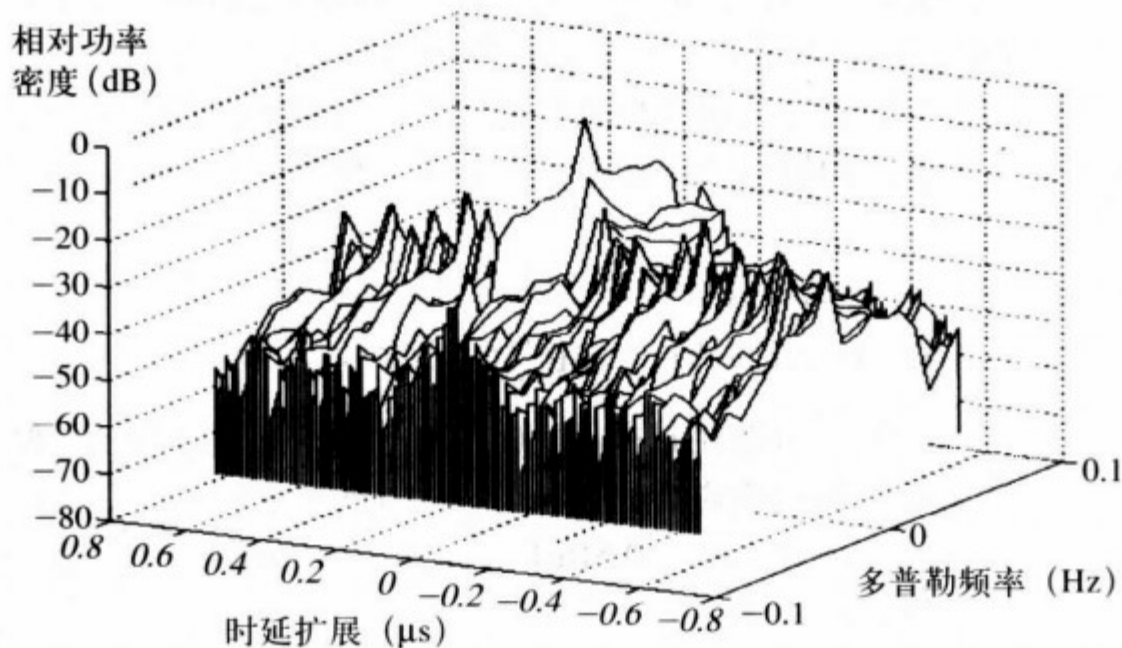
图3-12 散射函数
