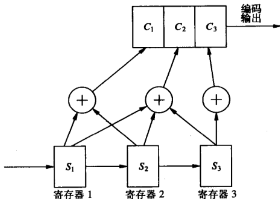
图8-24 题8.14和题8.15中的卷积码编码器
