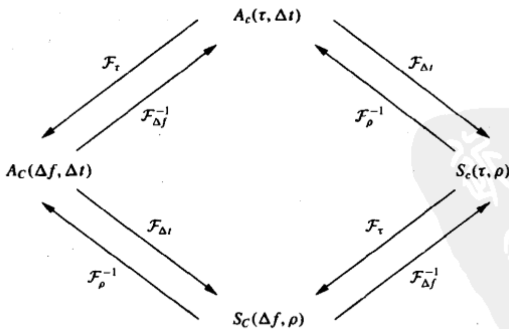
图3-15 傅里叶变换关系
