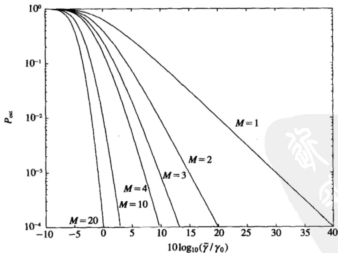
图7-2 瑞利衰落下选择合并的中断率
