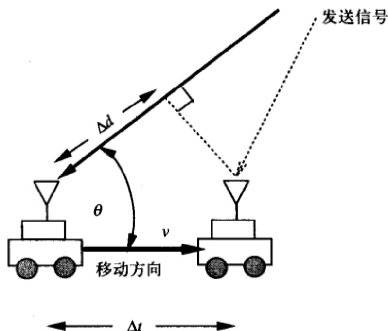
图2-2 多谱勒频移中的几何关系
