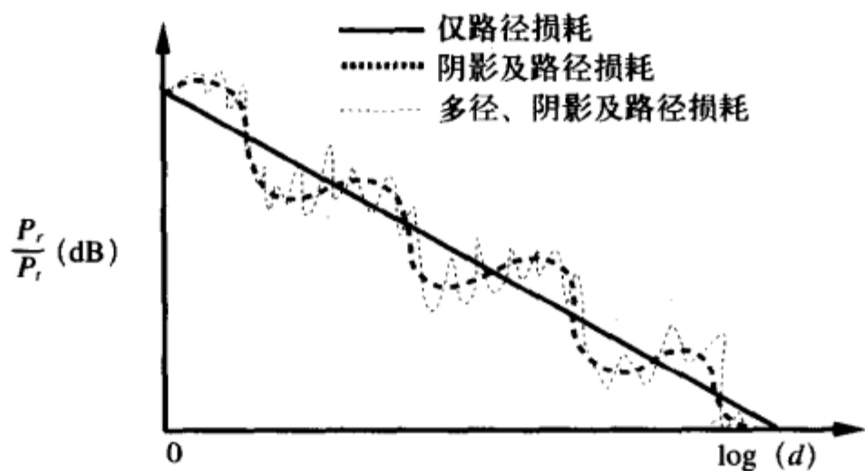
图2-1 路径损耗、阴影及多径与距离的关系
