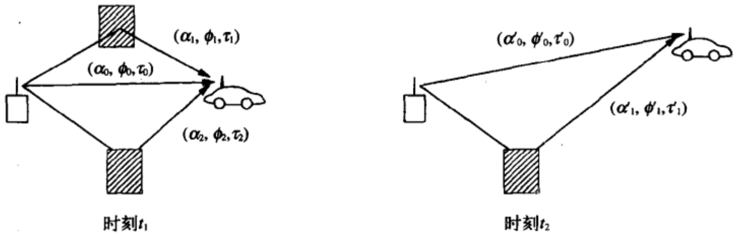
图3-2 不同观测时刻的多径情形
