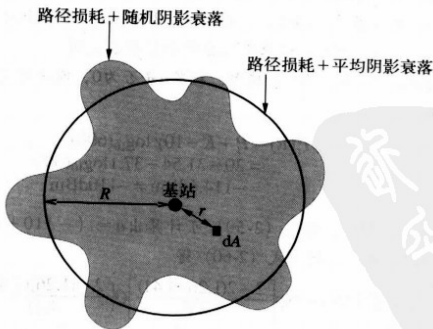
图2-10 等接收功率线
