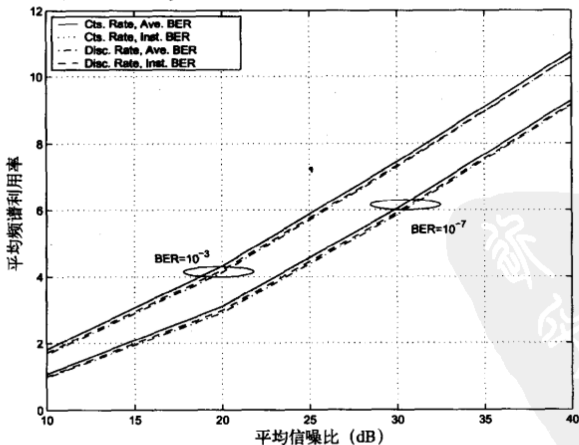
图9-16 不同自适应约束下的频谱利用率
