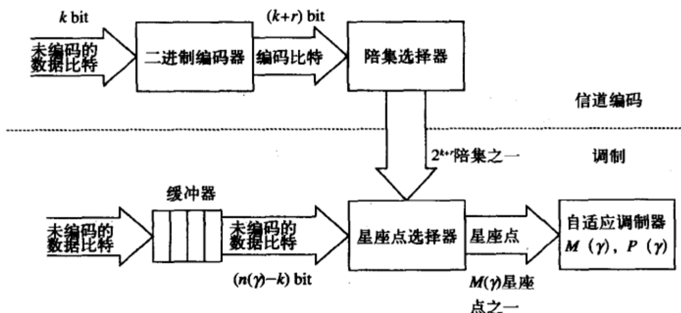
图9-13 自适应编码调制
